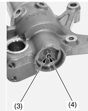
(3) válvulas de aire (4) centro de la válvula de aire de la cámara de equilibrio
