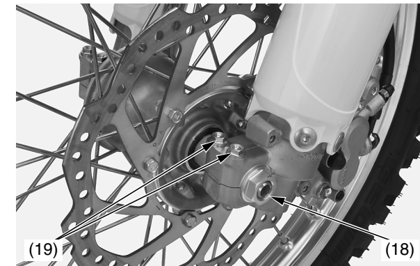
(18) tuerca del eje delantero (19) pernos de fijación del eje izquierdo
