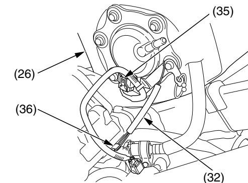
(26) depósito de combustible (32) cable del tope (35) conector B de la bomba de combustible (36) gancho del bastidor
