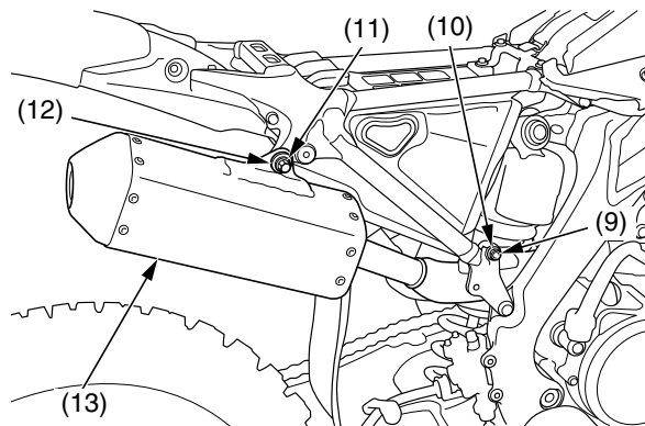
(9) perno A de montaje del silenciador derecho (10) arandela A (11) perno B de montaje del silenciador derecho (12) arandela B (13) silenciador derecho
