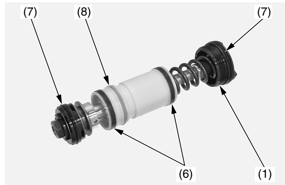
(1) conjunto de la tapa de la horquilla (6) bujes de la tapa de la horquilla (7) juntas tóricas (nuevas) (8) segmento de pistón
