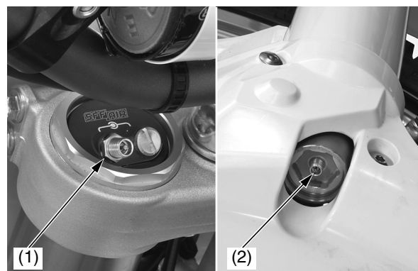
(1) válvula de aire de la cámara interior (2) válvula de aire de la cámara de equilibrio
