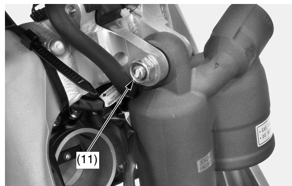
(11) tuerca superior del amortiguador trasero y perno
