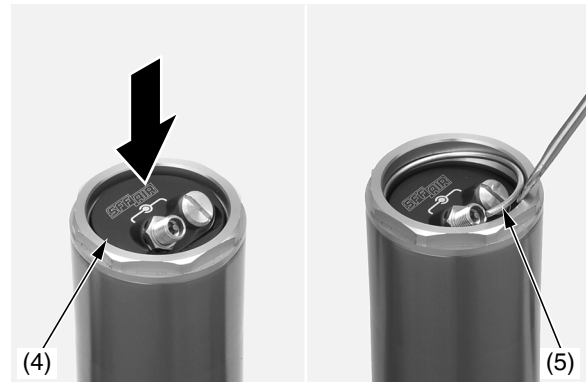
(4) tapa de la horquilla
