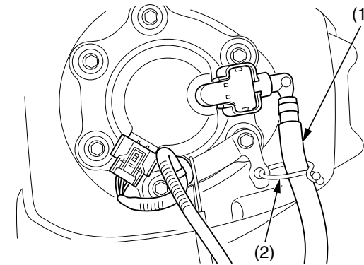
(1) manguera de suministro de combustible (2) abrazadera
