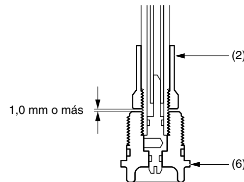
(2) contratuerca del perno central de la horquilla (6) perno central de la horquilla
