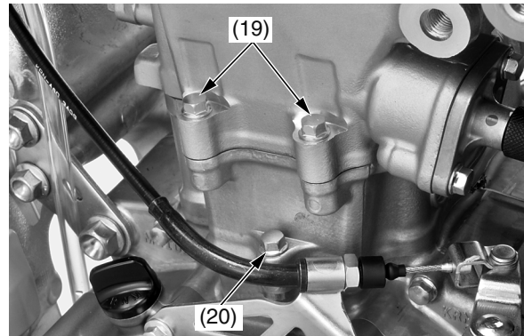
(19) pernos A de la culata (20) perno del cilindro
