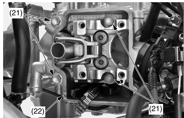
(21) pernos B y arandelas de la culata (22) culata
