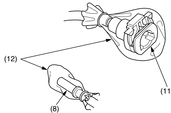
(8) juntas de combustible (11) conectores desconectados (12) bolsas de plástico
