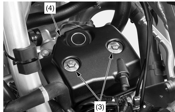
(3) pernos de la cubierta de la culata de cilindros y sellos de goma (4) cubierta de la culata
