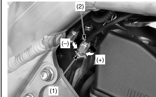
(1) contratuerca (+) aumentar el juego libre (2) ajustador (–) reducir el juego libre
