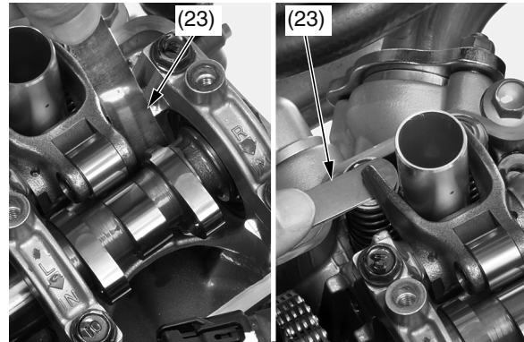
(23) juego de galgas
