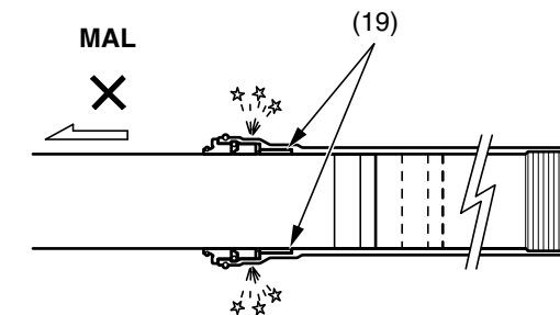
(19) bujes de la guía
