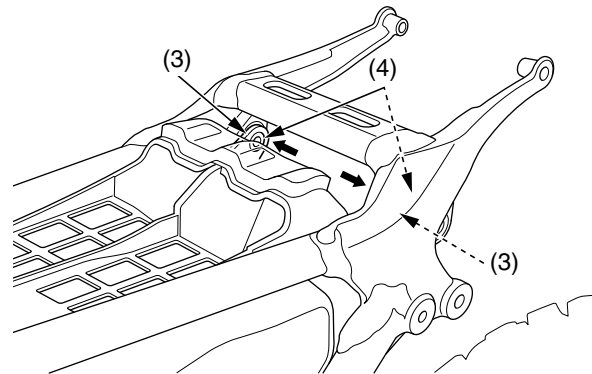
(3) caja del filtro de aire (4) bujes del bastidor secundario
