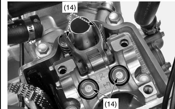
(14) laminillas de las válvulas
