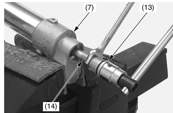
(7) soporte del eje (13) perno central de la horquilla (14) contratuerca del perno central de la horquilla
