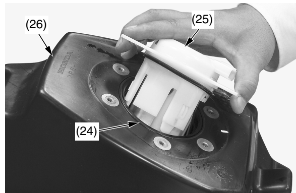
(24) junta tórica (nueva) (25) unidad de la bomba de combustible (26) depósito de combustible
