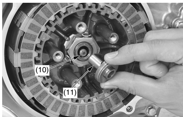
(10) barra del alzador del embrague (11) conjunto del alzador del embrague
