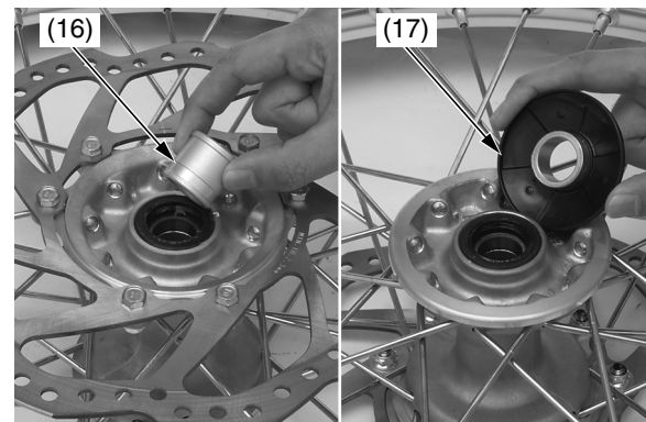
(16) collar del lado izquierdo (17) collar del lado derecho
