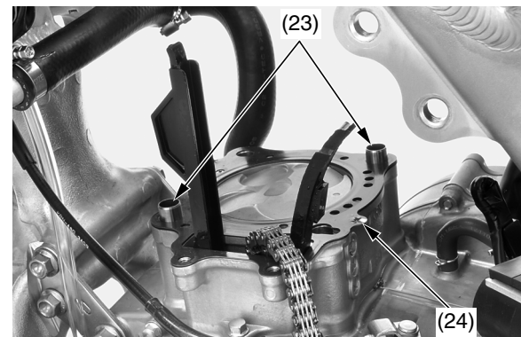
(23) pasadores cónicos (24) empaquetadura de la culata
