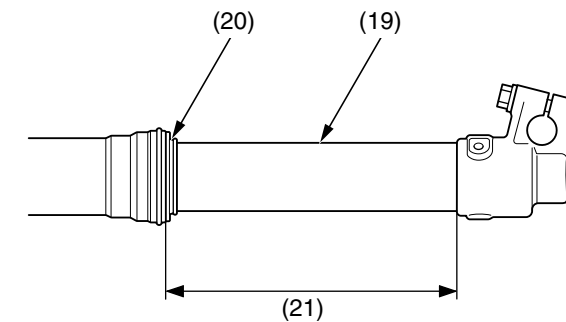
(19) superficie de deslizamiento (20) sello contra el polvo de la horquilla (21) longitud
