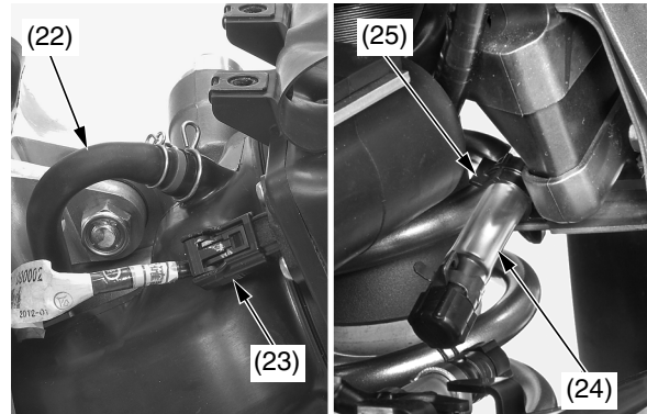
(22) tubo del respiradero A (23) Conector del sensor de IAT (24) tubo del respiradero B (25) retenedor
