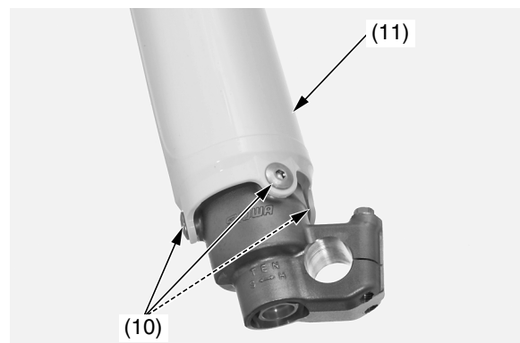
(10) pernos de cabeza hueca de los protectores de la horquilla (11) protector de la horquilla
