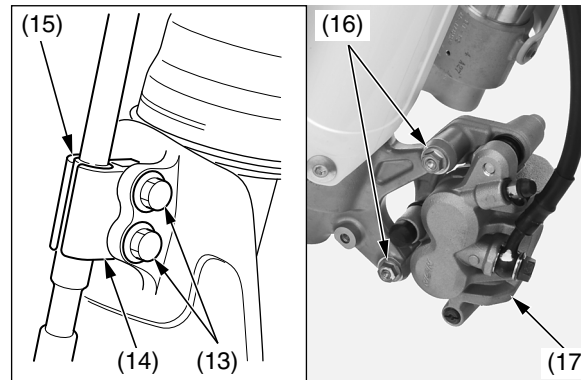
(13) pernos de la abrazadera de la manguera del freno (14) soporte A (15) soporte B (16) pernos de montaje de la pinza del freno delantero (17) pinza del freno
