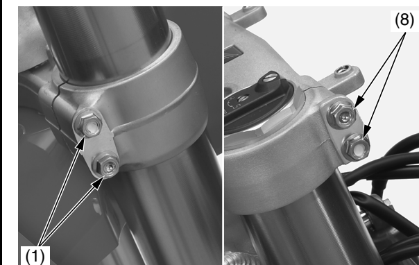
(1) pernos de fijación inferiores del puente de la horquilla (8) pernos de fijación superiores del puente de la horquilla
