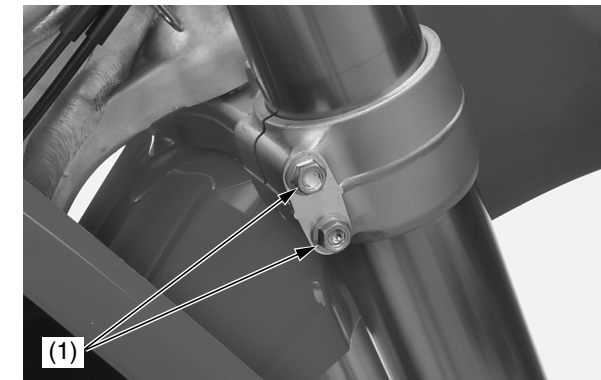
(1) pernos de fijación inferiores del puente de la horquilla
