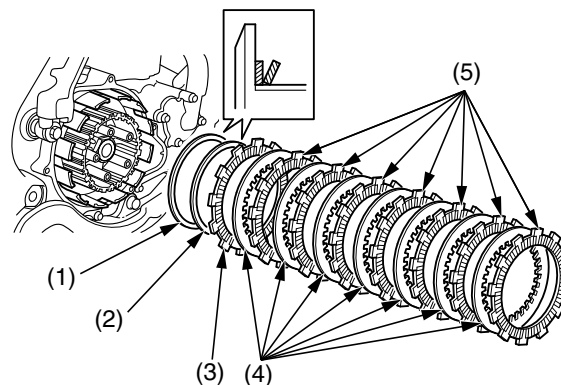
(1) asiento del resorte (2) resorte de trepidación (3) disco A del embrague (4) placas del embrague (5) discos B del embrague
