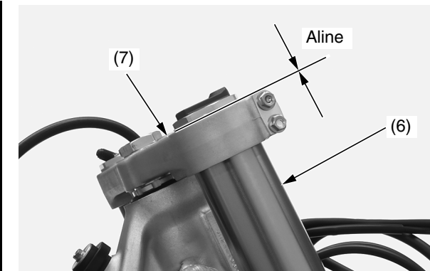
(6) tubo exterior (7) puente de la horquilla superior
