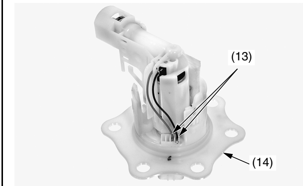
(13) terminales de los cables de la bomba de combustible (14) base de la bomba de combustible
