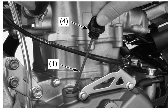
(1) tapa de relleno/varilla de medición del nivel de aceite de motor (4) junta tórica
