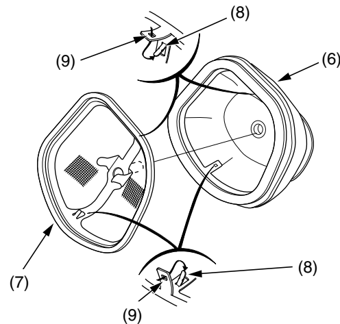
(6) elemento del filtro de aire (8) lengüetas del soporte (7) soporte del filtro de aire (9) orificios
