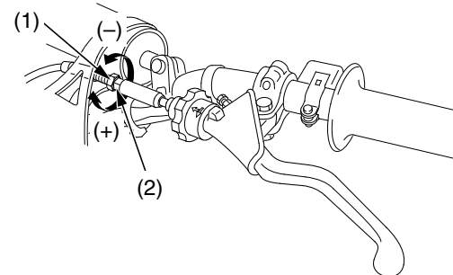
(1) contratuerca (2) ajustador del cable integral (+) aumentar el juego libre (–) reducir el juego libre
