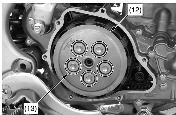
(12) placa de presión del embrague (13) resortes y pernos del embrague
