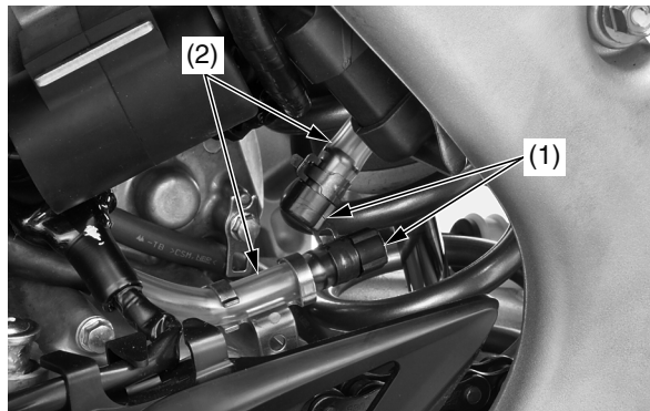
(1) tapones de los tubos del respiradero del cárter (2) tubos del respiradero del cárter
