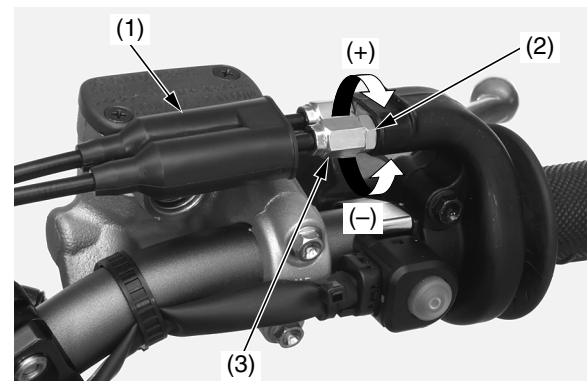
(1) cubierta contra el polvo (+) aumentar el juego libre (2) contratuerca (–) reducir el juego libre (3) ajustador
