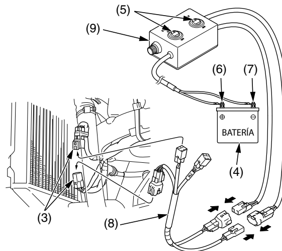
(3) conectores del mazo de cables secundario de DLC/ bomba de combustible (4) batería de 12 V (5) selectores del mazo de cables de la batería (6) cable positivo (+) del mazo de cables de la batería (7) cable negativo (-) del mazo de cables de la batería (8) adaptador del mazo de cables de la batería (9) mazo de cables de la batería
