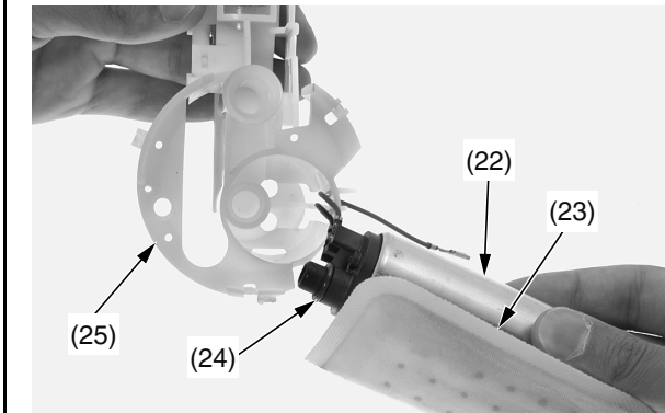
(22) conjunto de la bomba de combustible (23) filtro de la bomba de combustible (24) junta tórica (25) soporte de la unidad de la bomba de combustible
