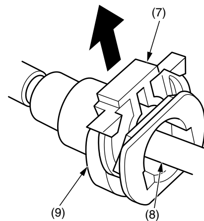
(7) retenedor de corredera (8) junta de combustible (9) caja del conector
