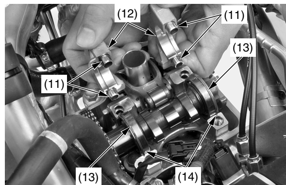
(11) pasadores cónicos (12) soportes del árbol de levas (13) anillos de ajuste (14) ranuras del cojinete del árbol de levas
