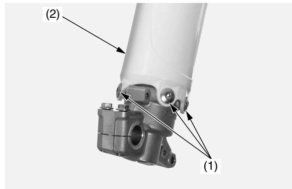
(1) pernos de cabeza hueca de los protectores de la horquilla (2) protector de la horquilla
