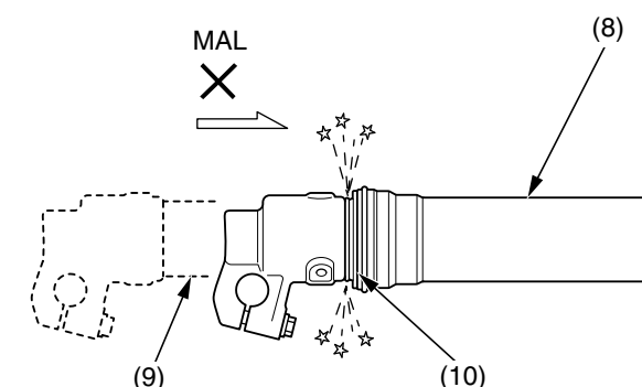
(8) tubo exterior (9) corredera (10) sello contra el polvo de la horquilla
