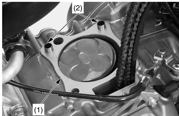
(1) empaquetadura del cilindro (nueva) (2) pasadores cónicos
