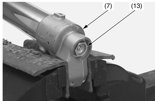
(7) soporte del eje (13) perno central de la horquilla
