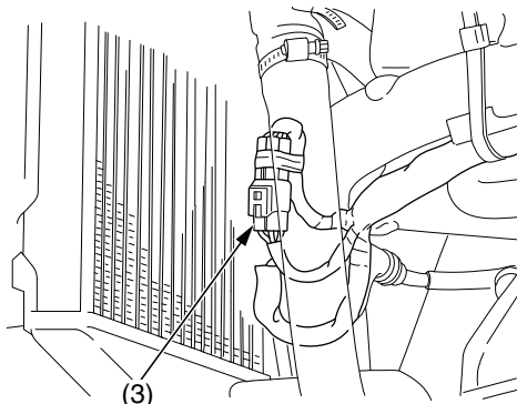
(3) conector del mazo de cables secundario de DLC/ bomba de combustible
