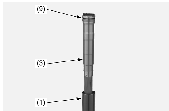
(1) conjunto de la horquilla (3) conjunto del amortiguador de la horquilla (9) junta tórica (nueva)
