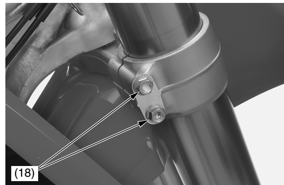
(18) pernos de fijación inferiores del puente de la horquilla
