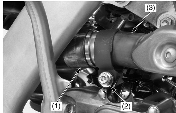
(1) empaquetadura (nueva) (2) abrazadera del silenciador derecho (3) tubo de escape
