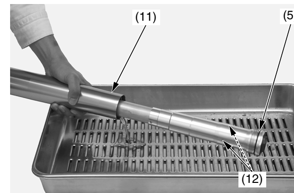
(5) amortiguador de la horquilla (11) tubo exterior/corredera (12) orificios de aceite
