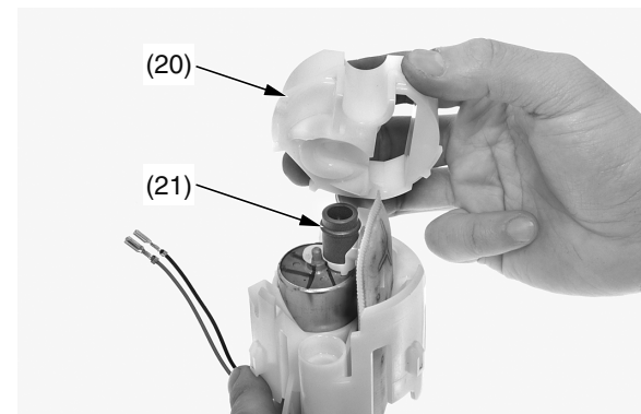
(20) tope de la bomba de combustible (21) goma amortiguadora
