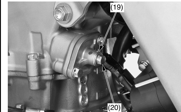
(19) arandela de sellado (nueva) (20) perno de la cubierta del alzador del tensor de la cadena de levas
