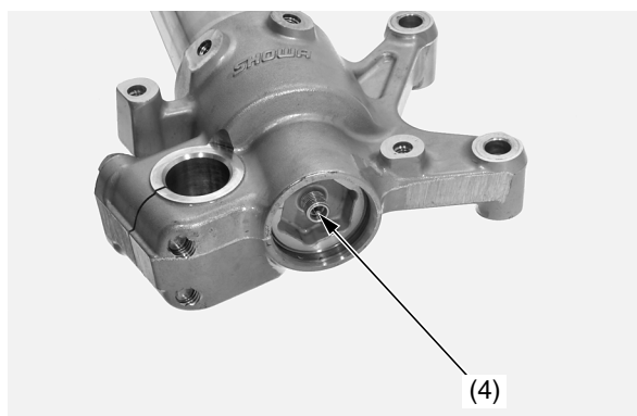
(4) centro de la válvula de aire de la cámara de equilibrio
