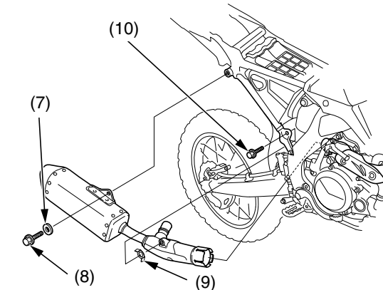
(2) abrazadera del silenciador derecho (4) silenciador derecho (5) lengüeta (6) corte (7) arandela B (8) perno B de montaje del silenciador derecho (9) arandela A (10) perno A de montaje del silenciador derecho
