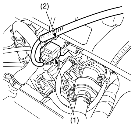
(1) conector A de la bomba de combustible (2) soporte
