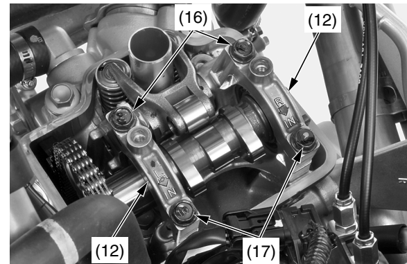
(12) soportes del árbol de levas (16) pernos A del soporte del árbol de levas (17) pernos B del soporte del árbol de levas
