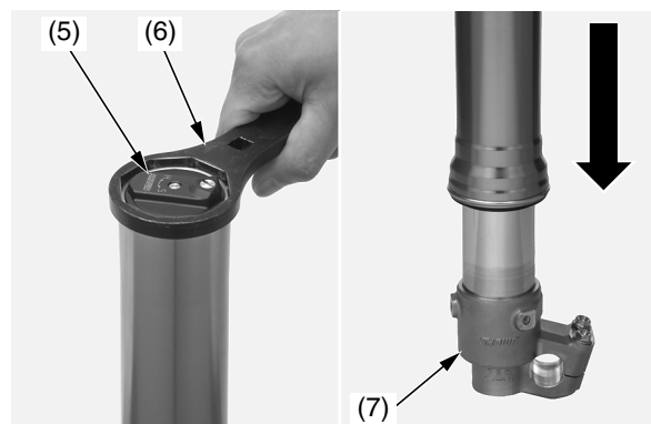
(5) amortiguador de la horquilla (6) llave de contratuercas (7) soporte del eje
