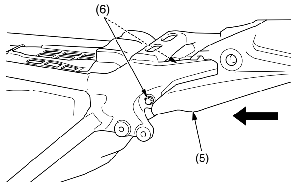
(5) guardabarros trasero (6) pernos de montaje y tuercas del guardabarros trasero
