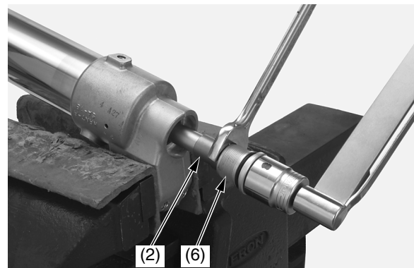
(2) contratuerca del perno central de la horquilla (6) perno central de la horquilla
