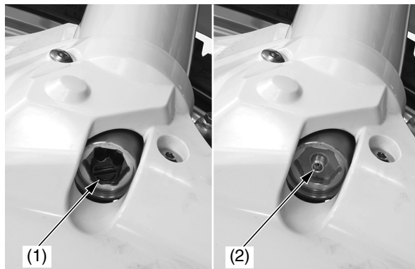
(1) tapón de la válvula (2) válvula de aire de la cámara de equilibrio
