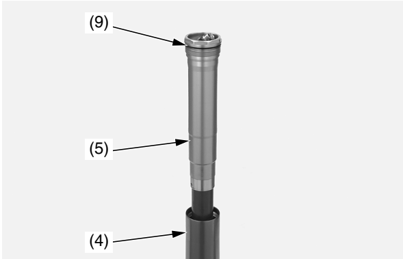
(4) tubo exterior (5) unidad de cilindro de aire (9) junta tórica
