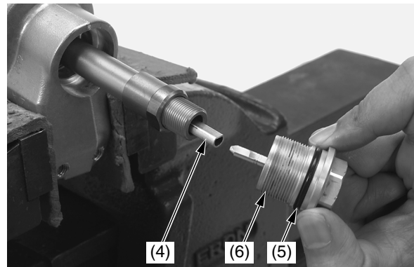
(4) varilla de empuje (5) junta tórica (nueva) (6) perno central de la horquilla
