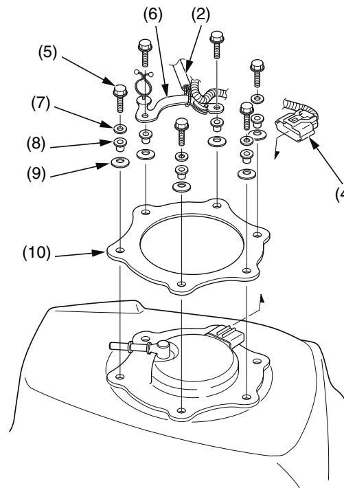
(2) cable del tope (4) conector B de la bomba de combustible (5) pernos de montaje de la bomba de combustible (6) guía del cable del tope (7) arandelas (8) collares (9) arandelas de resorte cónicas (10) placa de la bomba de combustible
