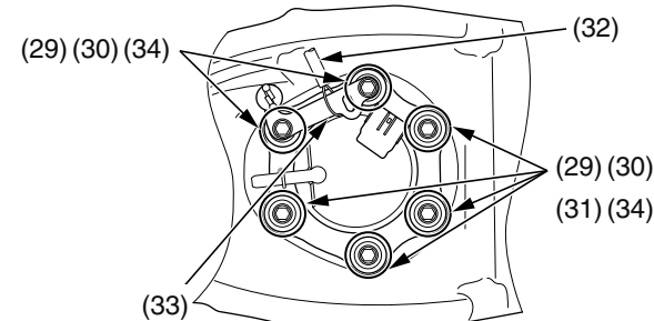
(29) arandelas de resorte cónicas (30) collares (31) arandelas (32) cable del tope (33) guía del cable del tope (34) pernos de montaje de la bomba de combustible
