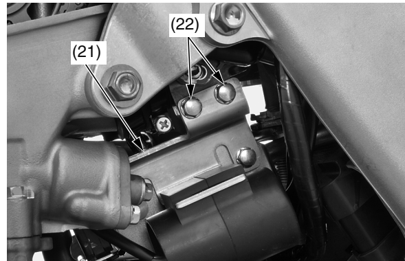
(21) soporte del condensador (22) pernos de montaje del soporte del condensador
