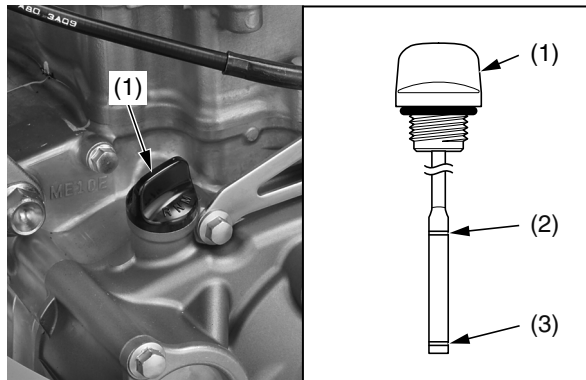
(1) tapa de relleno/varilla de medición del nivel de aceite de motor (2) marca de nivel superior (3) marca de nivel inferior
