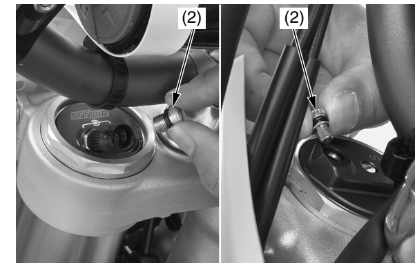
(2) tornillos de liberación de la presión
