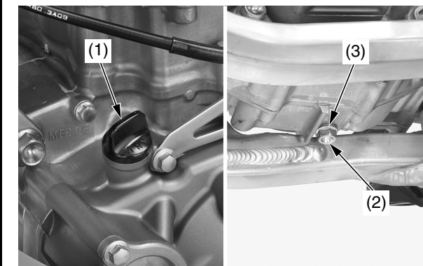
(1) tapa de relleno/varilla de medición del nivel de aceite de motor (2) Perno de drenaje de aceite de motor (3) arandela de sellado (nueva)
