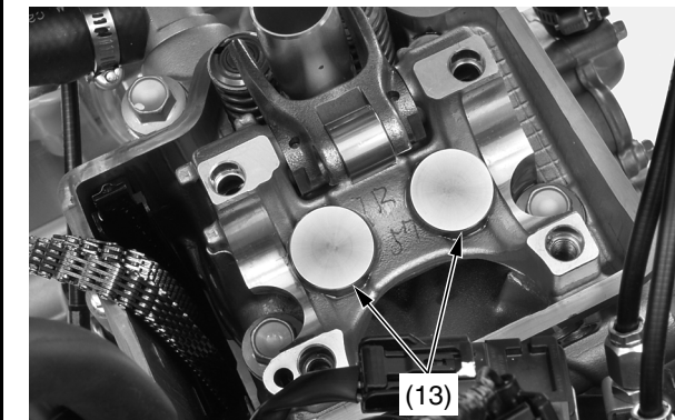
(13) alzaválvulas de admisión
