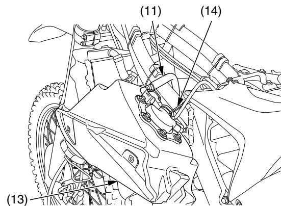
(11) manguera de suministro de combustible (13) depósito de combustible (14) cable de tope del depósito de combustible
