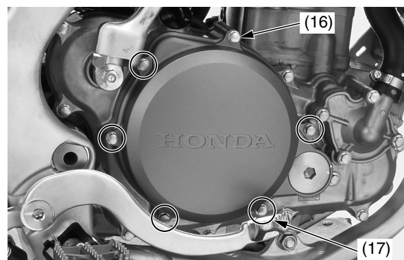
(16) perno A de la cubierta del embrague (17) pernos B de la cubierta del embrague
