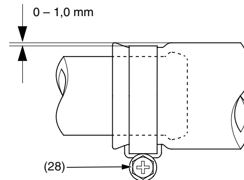
(28) tornillo de la abrazadera de la manguera del radiador
