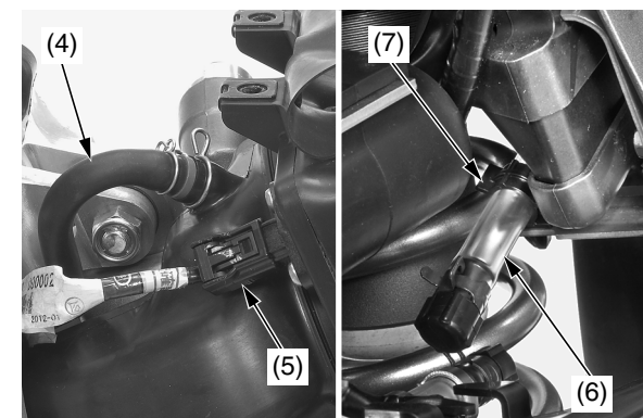
(4) tubo A del respiradero del cárter (5) Conector del sensor de IAT (6) tubo B del respiradero del cárter (7) retenedor
