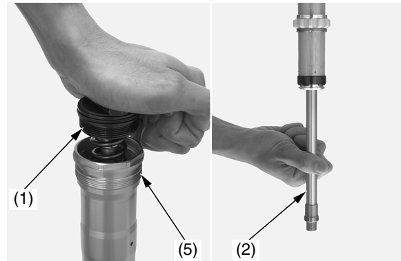
(1) conjunto de la tapa de la horquilla (2) barra del pistón del amortiguador de la horquilla (5) amortiguador de la horquilla
