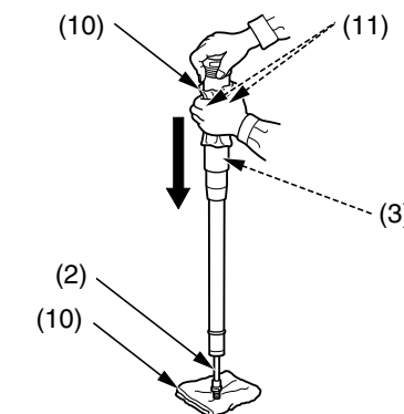
(2) barra del pistón del amortiguador de la horquilla (3) cámara de aceite del amortiguador de la horquilla (10) paño de taller (11) orificios de aceite
