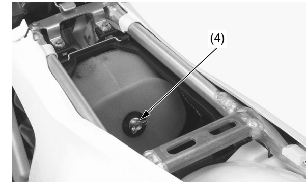
(4) perno de retención del filtro de aire
