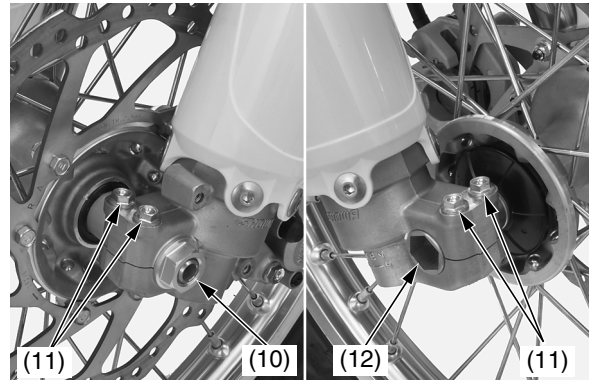
(10) tuerca del eje delantero (12) semieje delantero (11) pernos de fijación del eje
