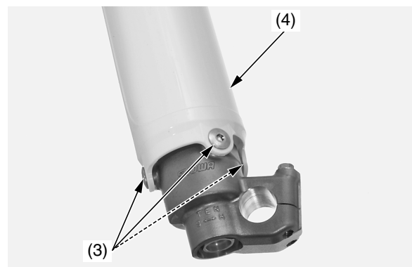
(3) pernos de cabeza hueca de los protectores de la horquilla (4) protector de la horquilla
