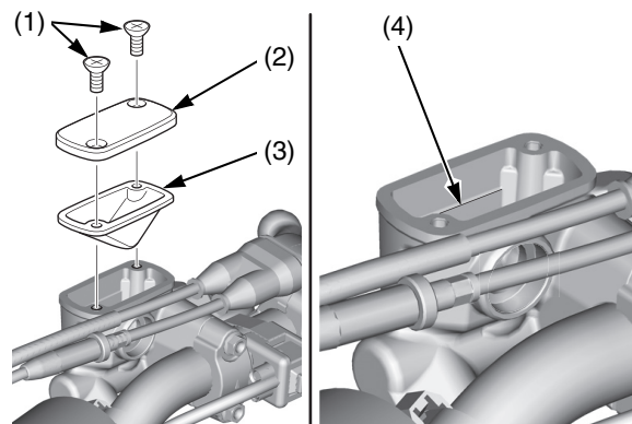
(1) viti del tappo del serbatoio del freno anteriore (2) tappo del serbatoio (3) diaframma (4) segno di livello superiore
