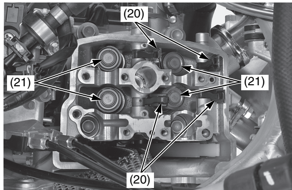
(20) bilancieri (21) spessori
