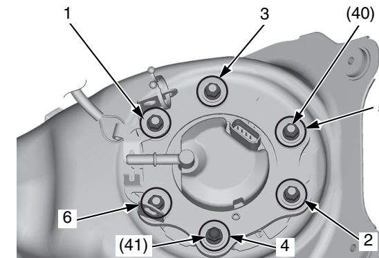
(40) dadi di fissaggio della pompa del carburante (41) dado cieco di fissaggio della pompa del carburante
