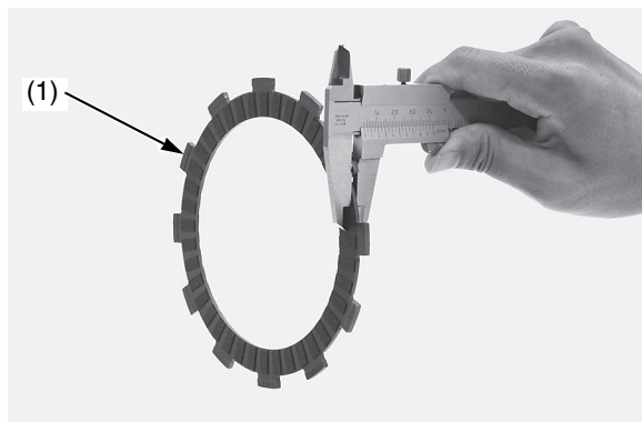
(1) disco conduttore della frizione
