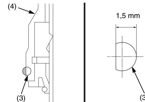
(3) anello di usura
