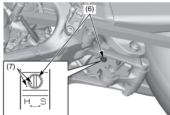
(6) registro dello smorzamento dell'estensione
