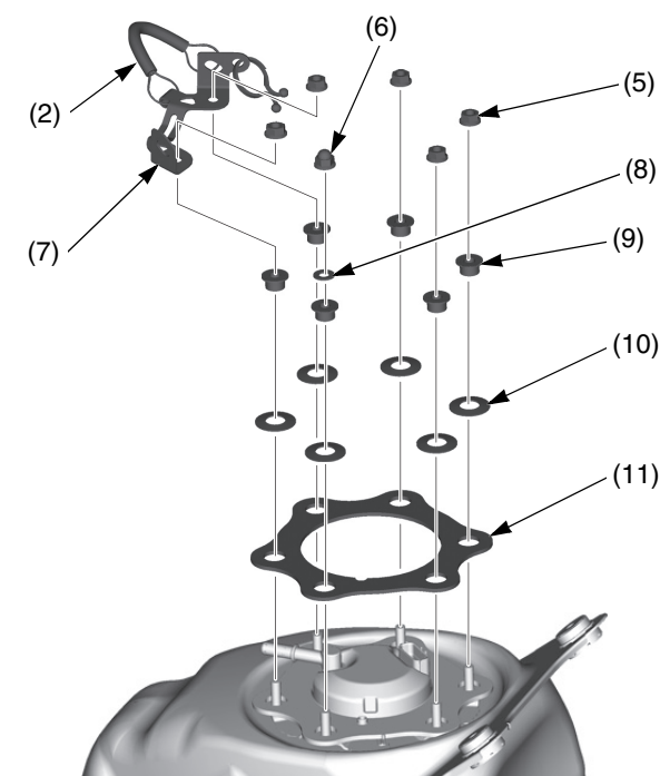
(2) cavo del fermo (5) dadi di fissaggio della pompa del carburante (6) dado cieco di fissaggio della pompa del carburante (7) guida del cavo del fermo (8) rondella (9) collari (10) rondelle elastiche coniche (11) piastra della pompa del carburante
