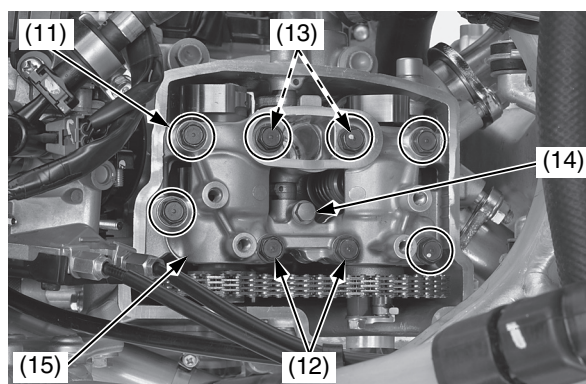
(11) bulloni A del supporto dell'albero a camme (12) bulloni B del supporto dell'albero a camme (13) rondelle (14) bullone di fermo dell'albero dei bilanciari (15) supporto dell'albero a camme
