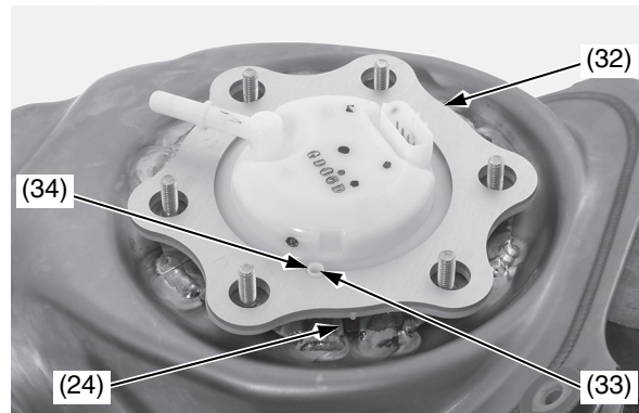
(24) sporgenza del parapolvere (32) piastra della pompa del carburante (33) scanalatura (34) sporgenza dell'unità della pompa del carburante
