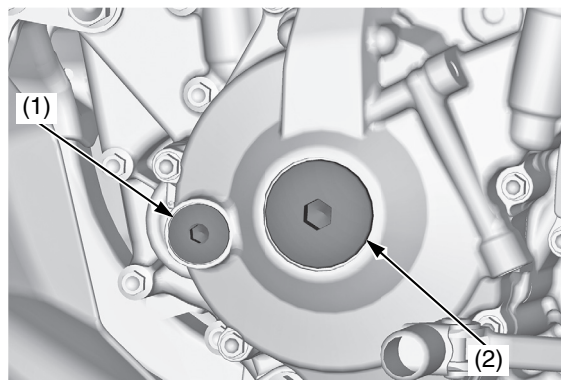
(1) tappo del foro di fasatura (2) tappo del foro dell'albero motore
