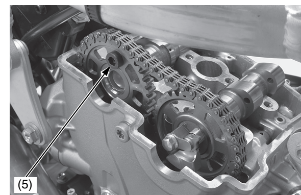
(5) bullone della corona della distribuzione
