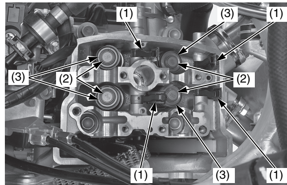
(1) bilancieri (3) fermi delle molle delle valvole (2) spessori delle valvole
