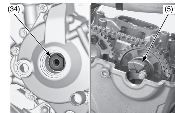
(5) peso del decompressore (34) volano
