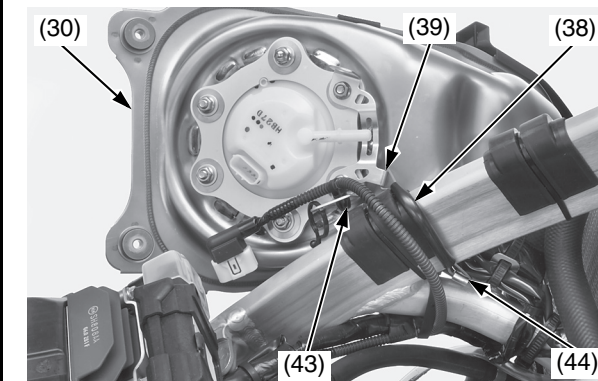
(30) serbatoio del carburante (38) cavo del fermo (39) guida del cavo del fermo (43) fermaglio della fascetta del cablaggio (44) gancio sul telaio
