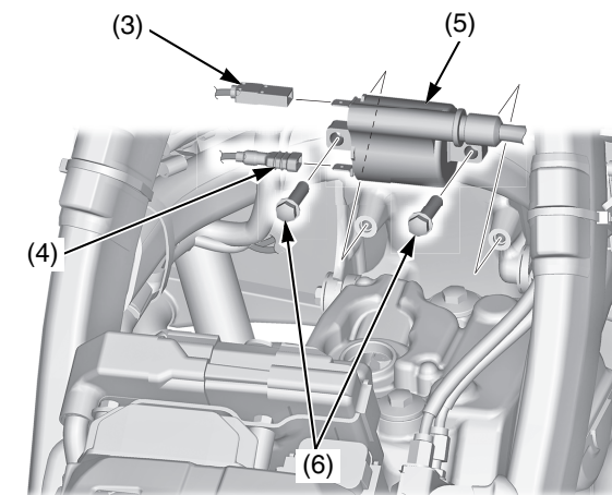
(3) connettore A della bobina di accensione (4) connettore B della bobina di accensione (5) bobina di accensione (6) bulloni della bobina di accensione
