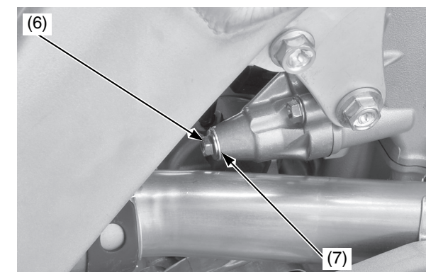
(6) bullone del coperchio del sollevatore del tenditore della catena di distribuzione
