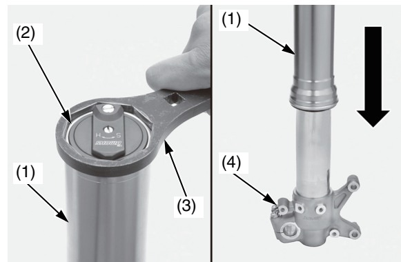
(1) tubo esterno (2) gruppo dell'ammortizzatore della forcella (3) chiave inglese (4) supporto dell'asse
