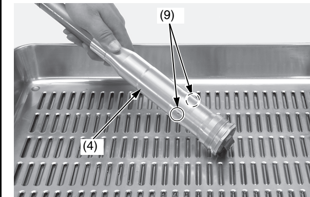
(4) gruppo dell'ammortizzatore della forcella (9) fori dell'olio
