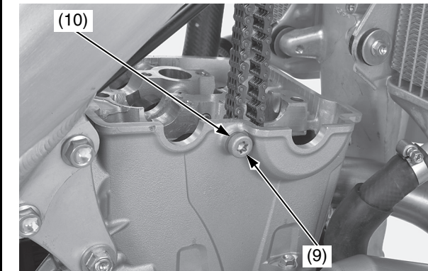
(9) bullone di tenuta (10) rondella di tenuta
