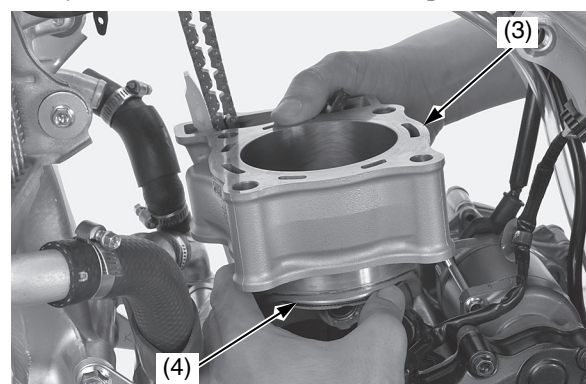
(3) cilindro (4) pistone
