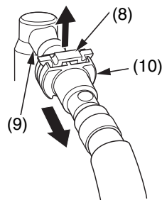
(8) fermo scorrevole (9) giunto del carburante (10) alloggiamento del connettore
