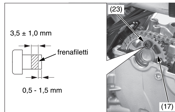
(17) corona della distribuzione di aspirazione (23) bullone della corona della distribuzione
