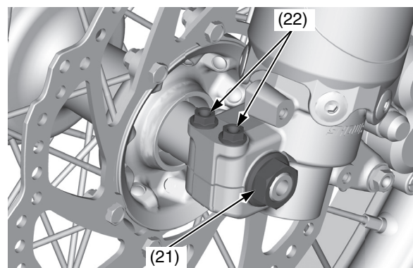
(21) dado del perno ruota anteriore (22) bulloni di fissaggio dell'asse sinistro
