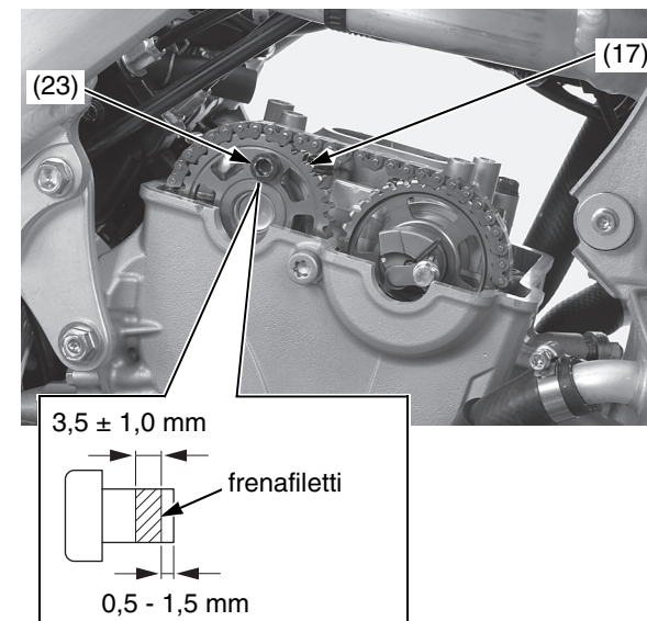
(17) corona della distribuzione di aspirazione (23) bullone della corona della distribuzione
