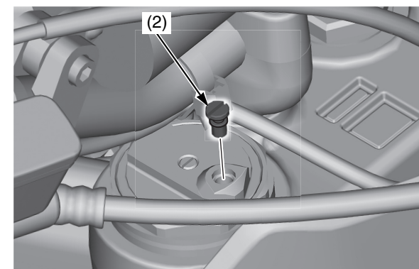
(2) viti di scarico della pressione dell'aria
