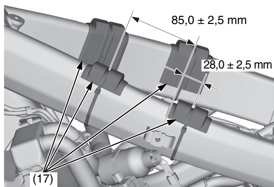
(17) tamponi di gomma
