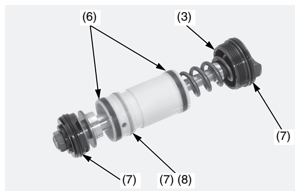
(3) gruppo bulloni della forcella (6) boccole dei bulloni della forcella (7) O-ring (nuovi) (7) (8) fascia elastica del pistone (nuova)
