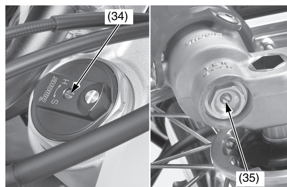
(34) registro dello smorzamento della compressione (35) registro dello smorzamento dell'estensione
