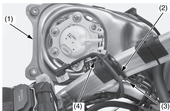
(1) serbatoio del carburante (2) cavo del fermo (3) gancio sul telaio (4) fermaglio della fascetta del cablaggio
