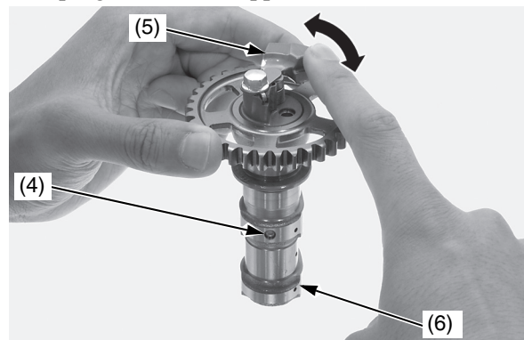
(4) stantuffo (6) albero a camme di scarico (5) peso del decompensatore
