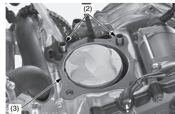
(2) perni di centraggio (3) guarnizione cilindro (nuova)
