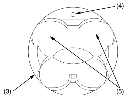
(3) pistone (5) incavi grandi delle valvole (4) segno "o"
