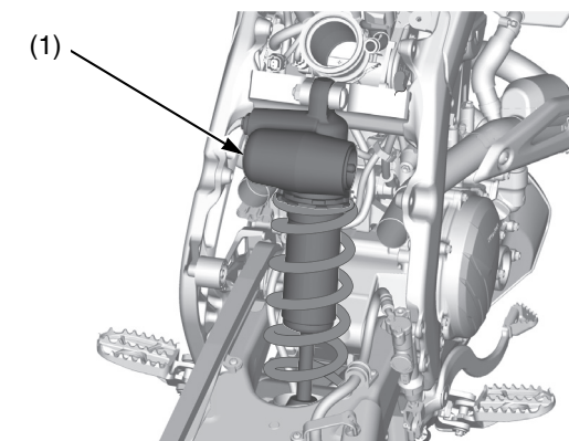
(1) ammortizzatore posteriore
