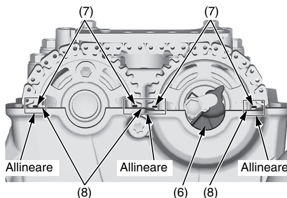
(6) peso del decompressore (7) segni della fasatura (8) superficie di accoppiamento della testata
