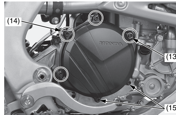
(13) rondella (nuova) (14) bulloni A del coperchio della frizione (15) bulloni B del coperchio della frizione
