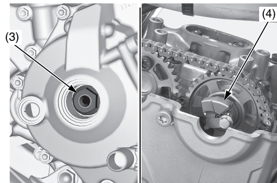
(3) volano
