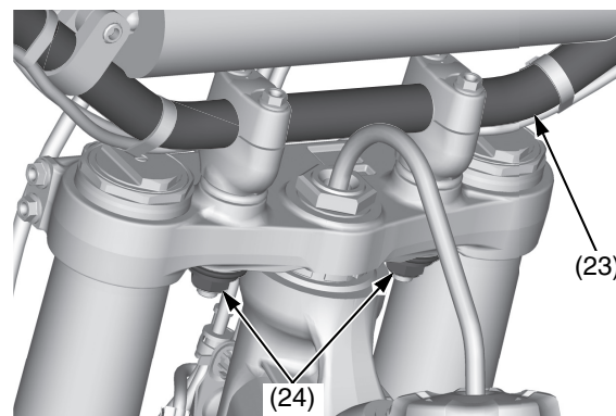
(23) manubrio (24) gommini di montaggio, rondelle e dadi dei supporti inferiori del manubrio
