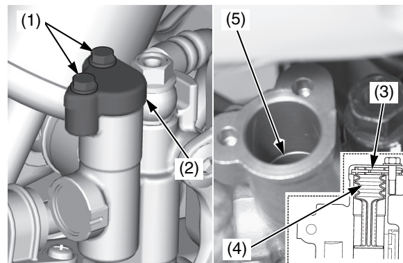
(1) bulloni del tappo del serbatoio del freno posteriore (2) tappo del serbatoio (3) piastra di fissaggio (4) diaframma (5) segno di livello superiore
