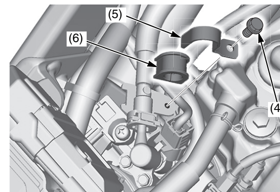
(4) bullone
