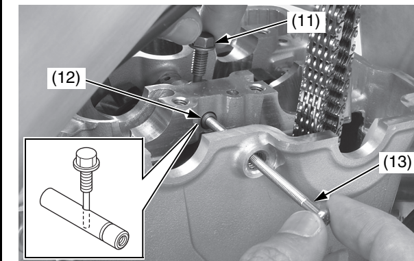
(11) bullone di fermo dell'albero dei bilancieri (12) albero dei bilancieri (13) bullone da 4 mm
