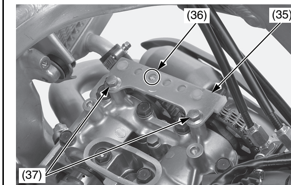
(35) guida della catena di distribuzione (37) bulloni della guida della catena di distribuzione (36) segno "⇐"
