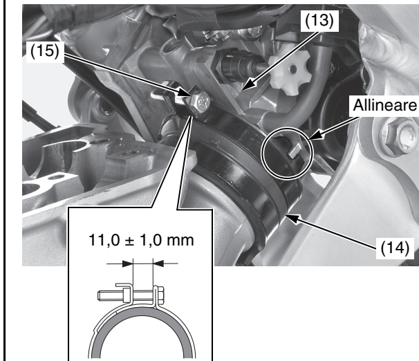
(13) corpo farfallato
