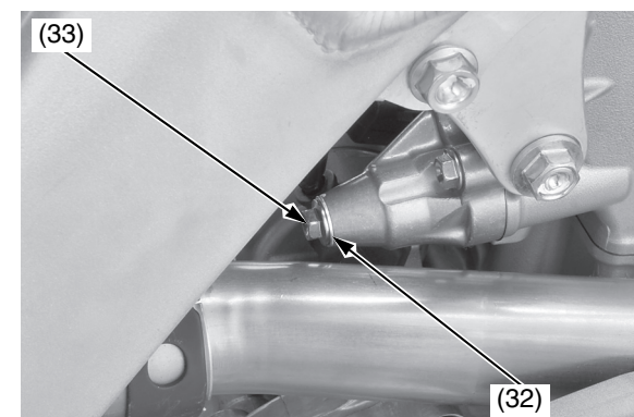
(32) rondella di tenuta (nuova) (33) bullone del coperchio del sollevatore del tenditore della catena di distribuzione
