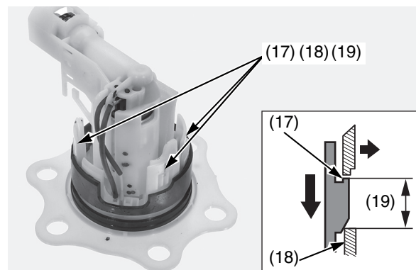
(17) ganci (18) linguette
