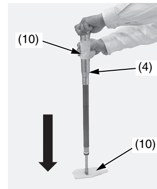
(4) gruppo dell'ammortizzatore della forcella (10) panni da officina
