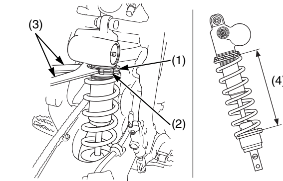
(1) dado di bloccaggio della molla dell'ammortizzatore (2) dado di registro
