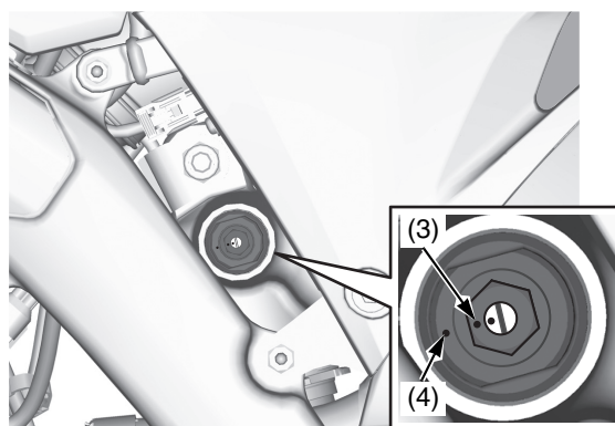
(3) segno punzonato sul registro dello smorzamento della compressione ad alta velocità (4) segno punzonato sul corpo del registro
