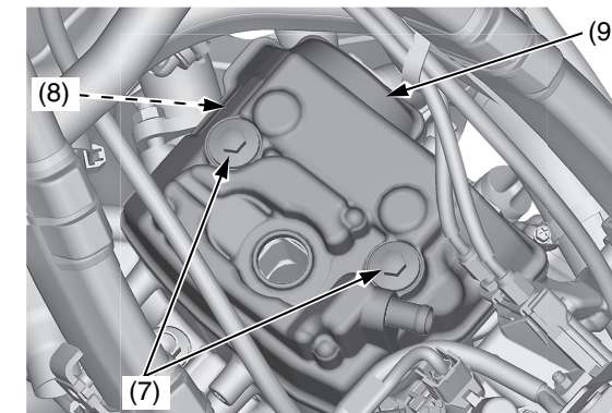
(7) bulloni a brugola del coperchio della testata, guarnizioni di gomma (8) guarnizione del coperchio della testata (9) coperchio della testata
