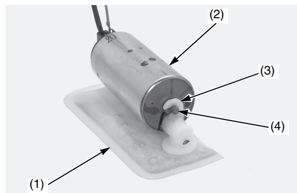
(1) filtro della pompa del carburante (2) gruppo della pompa del carburante (3) gancio (4) protuberanza di unione del carburante
