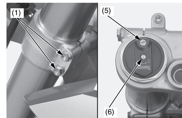
(1) bulloni di fissaggio inferiori del ponte della forcella (5) vite di scarico della pressione dell'aria (6) registro dello smorzamento della compressione
