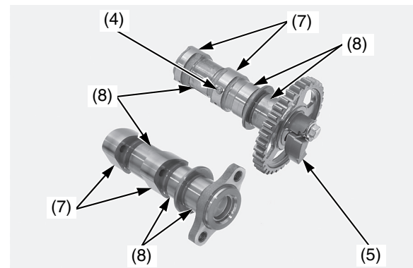
(4) stantuffo (5) peso del decompensatore (7) lobi delle camme dell'albero a camme (8) superfici del perno di banco
