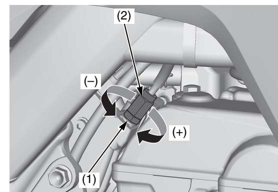
(1) dado di bloccaggio (2) registro
