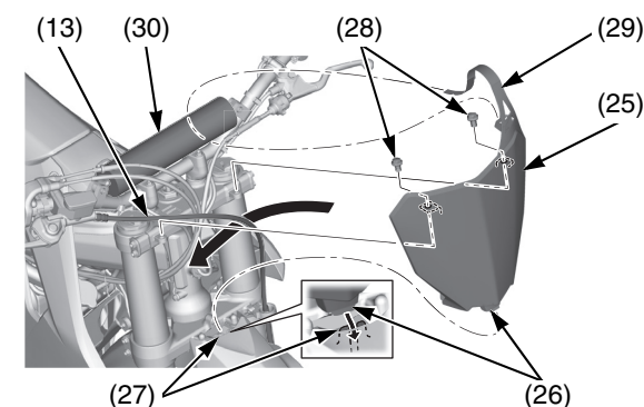
(13) tubo flessibile del freno (28) bulloni della targa (25) targa porta numero (29) linguetta della targa porta numero (26) linguetta (30) manicotto di protezione del manubrio (27) fessura
