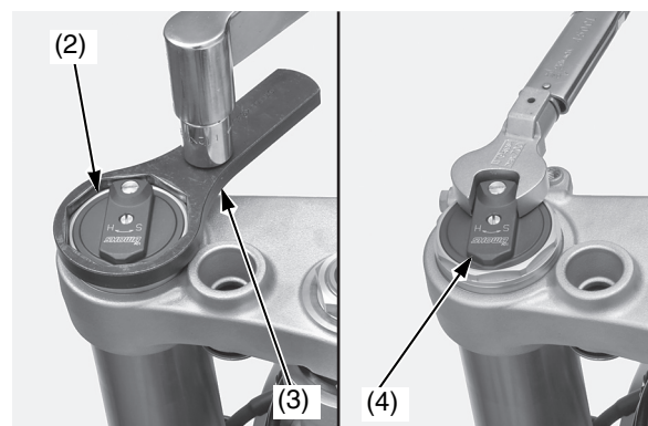
(2) gruppo dell'ammortizzatore della forcella (3) chiave inglese (4) gruppo bulloni della forcella
