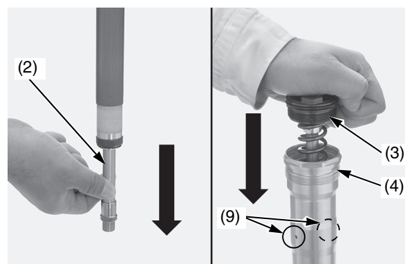
(2) asta dell'ammortizzatore forcella (3) gruppo bulloni della forcella (4) gruppo dell'ammortizzatore della forcella (9) fori dell'olio
