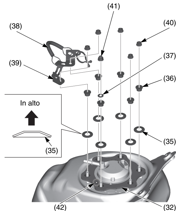
(32) piastra della pompa del carburante (35) rondelle elastiche coniche (36) collari (37) rondella (38) cavo del fermo (39) guida del cavo del fermo (40) dadi di fissaggio della pompa del carburante (41) dado cieco di fissaggio della pompa del carburante (42) segno identificativo
