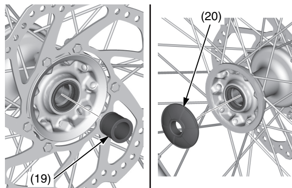
(19) collare sinistro
