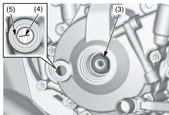
(3) volano (5) segno di riferimento (4) segno corrispondente
