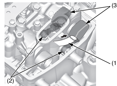
(1) spessore (3) lobi delle camme dell'albero a camme (2) bilancieri di aspirazione
