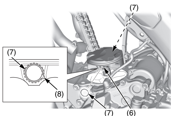
(6) spinotto del pistone (8) cavità del pistone (7) fermagli dello spinotto del pistone (nuovi)
