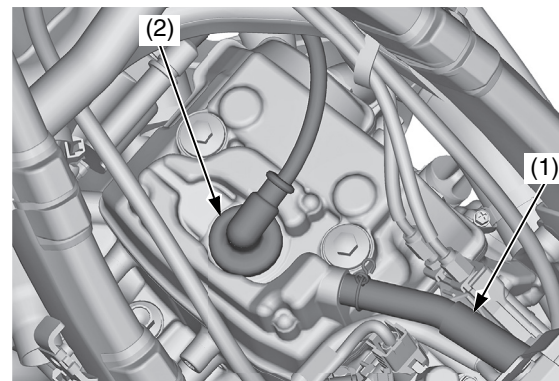
(1) tubo di sfiato
