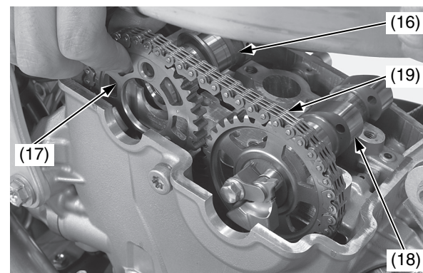
(16) albero a camme di aspirazione (17) corona della distribuzione di aspirazione (18) albero a camme di scarico (19) catena di distribuzione
