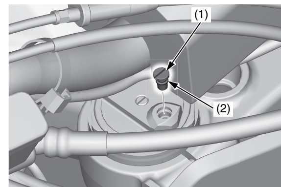
(1) vite di scarico della pressione (2) O-ring (nuovo) dell'aria
