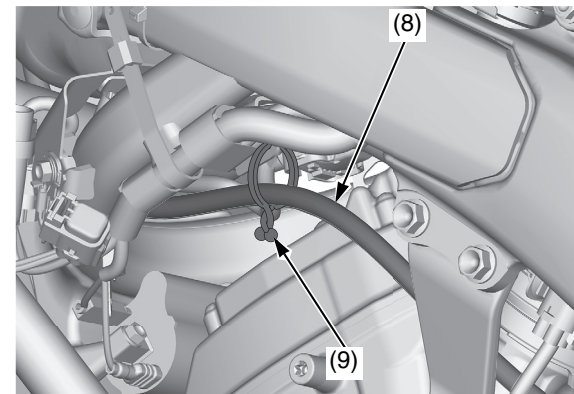
(8) tubo flessibile di trabocco (9) morsetto
