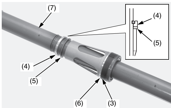
(3) boccola di scorrimento (4) fermo della sede (5) anello di sostegno (6) collare della sede della molla (7) pompante della forcella
