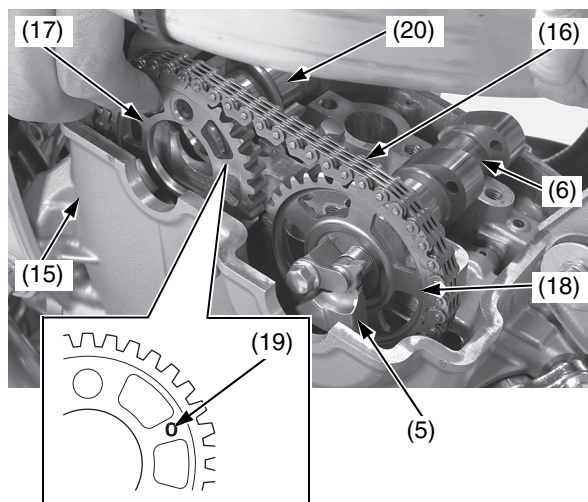
(5) peso del decompressore (6) albero a camme di scarico (15) testata (16) catena di distribuzione (17) corona della distribuzione di aspirazione (18) corona della distribuzione di scarico (19) segno "O"
