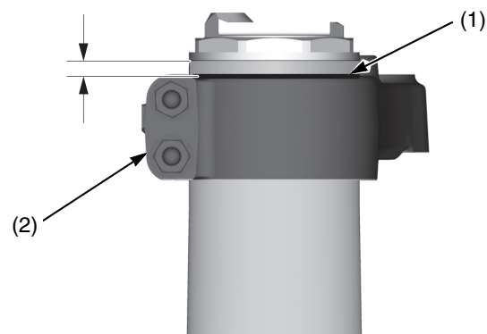
(1) scanalatura (2) ponte superiore della forcella
