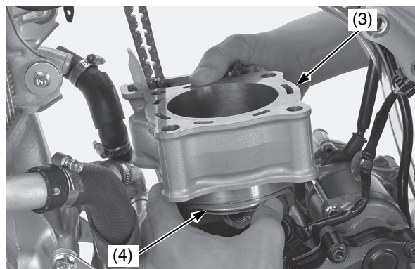
(3) cilindro (4) pistone
