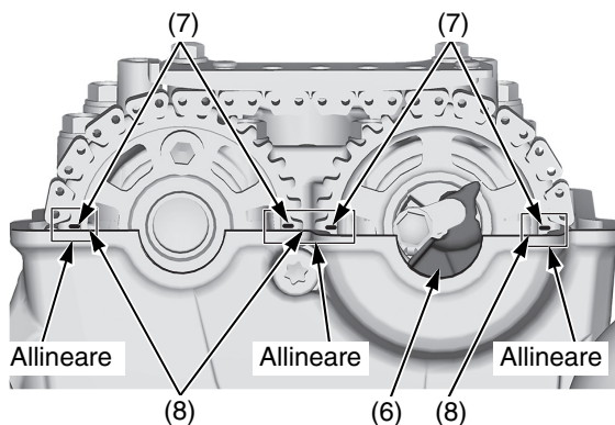
(6) peso del decompressore
