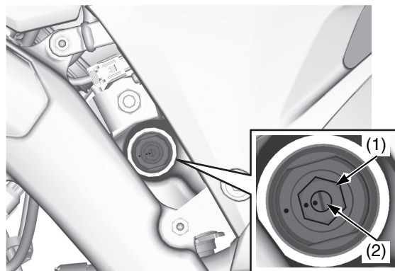
(1) registro dello smorzamento della compressione ad alta velocità (2) registro dello smorzamento della compressione a bassa velocità
