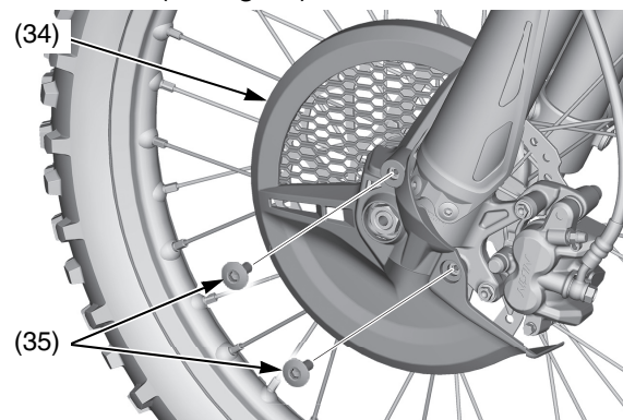
(34) coperchio del disco (35) bulloni a brugola del coperchio del disco
