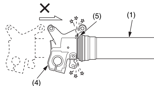
(1) tubo esterno (4) supporto dell'asse
