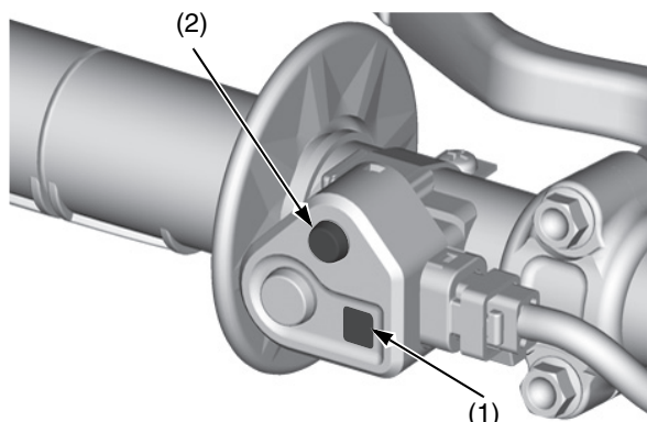
(1) spia del sistema di controllo lancio (viola) (2) pulsante di selezione settaggio motore
