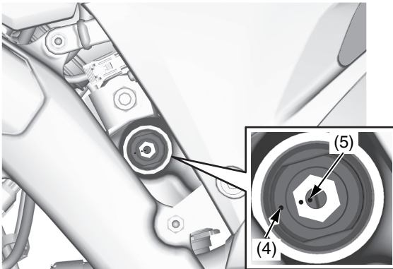
(4) segno punzonato sul corpo del registro (5) segno punzonato sul registro dello smorzamento della compressione a bassa velocità
