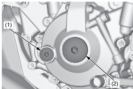
(1) tappo del foro di fasatura
