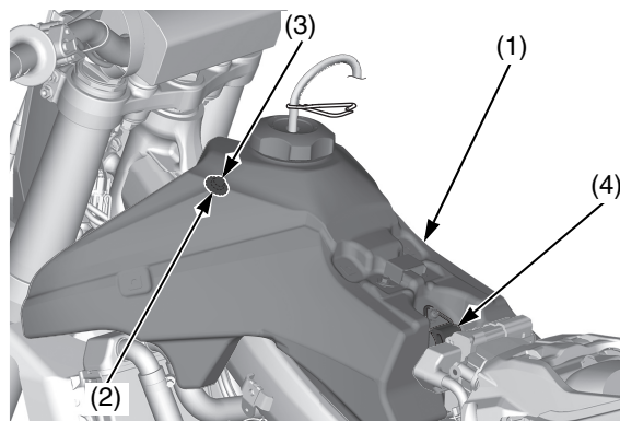
(1) serbatoio del carburante (2) collare (3) bullone del serbatoio carburante (4) fascia del serbatoio del carburante
