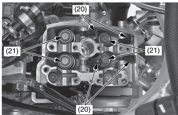
(20) bilanciери (21) spessori
