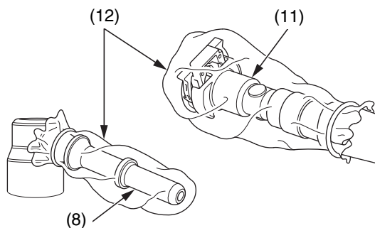
(8) giunto del carburante (11) connettore scollegato (12) sacchetti di plastica
