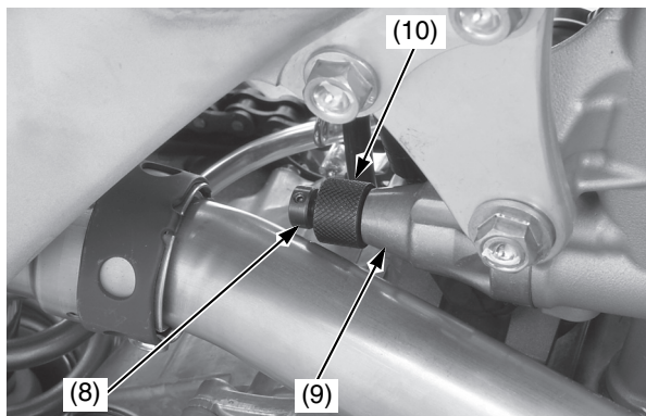
(8) attrezzo di blocco del tenditore (9) sollevatore del tenditore della catena di distribuzione (10) ghiera
