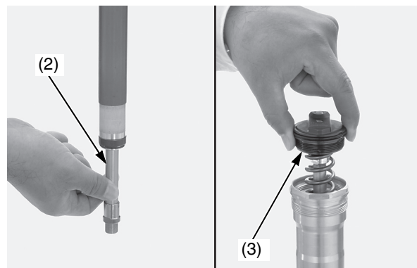
(2) asta del pompante forcella (3) gruppo bulloni della forcella
