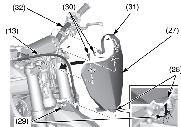
(13) tubo flessibile del freno (30) bulloni della targa (27) targa porta numero (31) linguetta della targa (28) linguetta porta numero (29) fessura (32) manubrio
