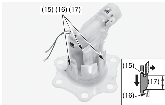
(15) ganci (16) linguette
