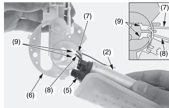
(2) gruppo della pompa del carburante (5) O-ring (nuovo) (6) supporto dell'unità della pompa del carburante (7) filo rosso (8) filo nero (9) scanalature
