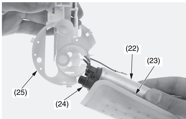
(22) gruppo della pompa del carburante (23) filtro della pompa del carburante (24) O-ring (25) supporto dell'unità della pompa del carburante
