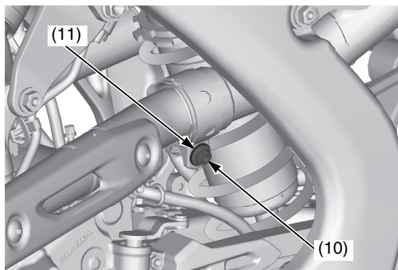
(10) bullone del morsetto (11) rondella del terminale di scarico sinistro
