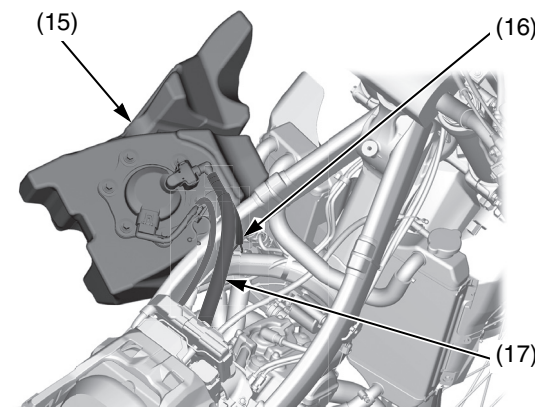
(15) serbatoio del carburante (16) cavo del fermo del serbatoio del carburante (17) tubo flessibile di alimentazione del carburante
