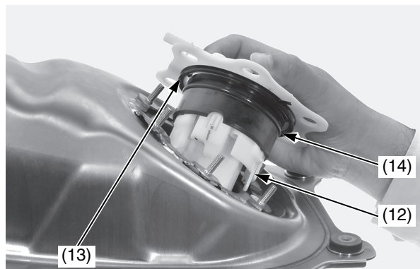
(12) unità della pompa del carburante (13) parapolvere (14) O-ring
