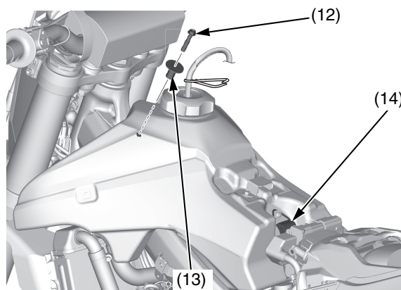
(12) bullone del serbatoio carburante (14) fascia del serbatoio del carburante (13) collare
