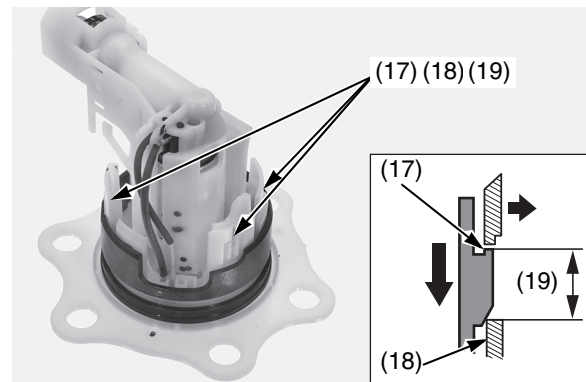
(17) ganci (18) linguette
