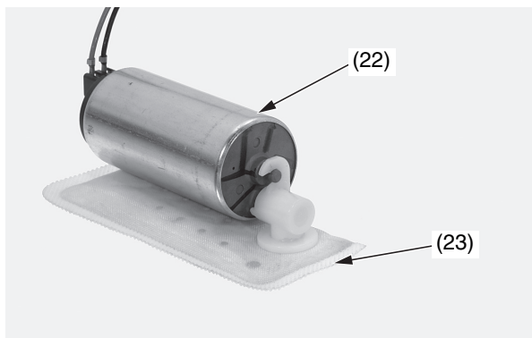
(22) gruppo della pompa del carburante (23) filtro della pompa del carburante
