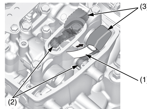
(1) spessimetro
