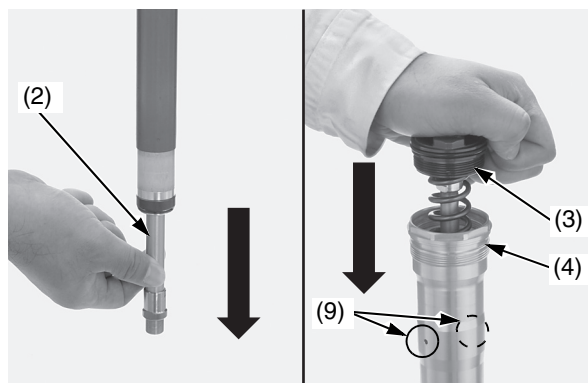
(2) asta del pompante forcella (3) gruppo bulloni della forcella (4) gruppo del pompante della forcella (9) fori dell'olio
