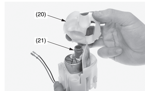
(20) fermo della pompa del carburante (21) tampone ammortizzatore
