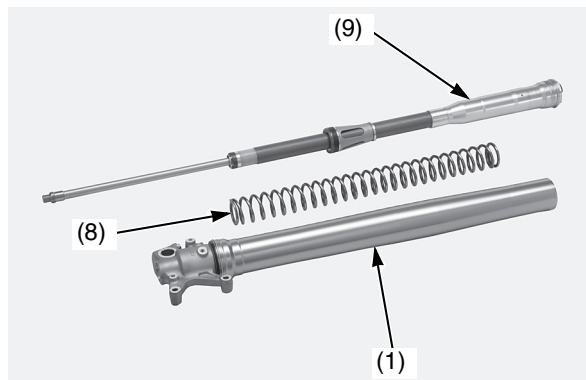
(1) gruppo della forcella (8) molla della forcella (9) gruppo del pompante della forcella
