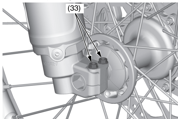
(33) bulloni di fissaggio dell'asse destro
