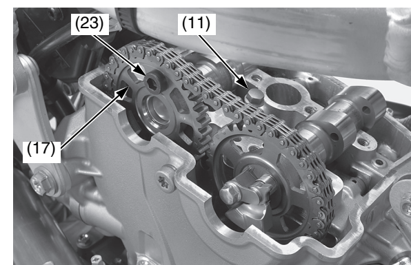
(11) bullone di fermo dell'albero dei bilancieri (17) corona della distribuzione di aspirazione (23) bullone della corona della distribuzione
