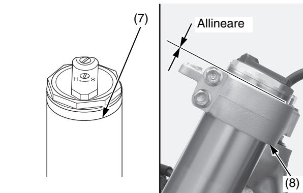
(7) scanalatura
