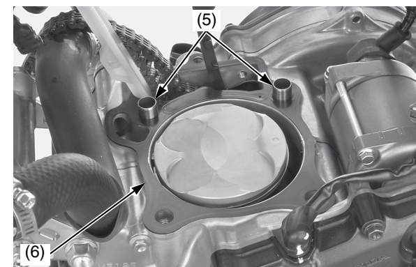
(5) perni di centraggio (6) guarnizione del cilindro
