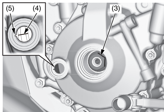
(3) volano
