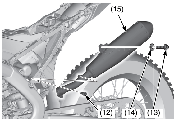
(12) bullone di fissaggio A del terminale di scarico sinistro (13) bullone di fissaggio B del terminale di scarico sinistro (14) rondella (15) terminale di scarico sinistro
