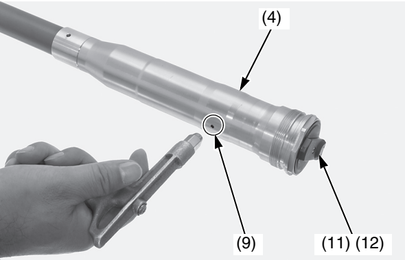
(4) gruppo del pompante della forcella (9) fori dell'olio (11) viti di scarico della pressione dell'aria (12) O-ring (nuovi)
