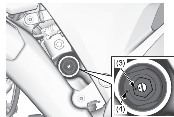
(3) segno punzonato sul registro dello smorzamento della compressione ad alta velocità (4) segno punzonato sul corpo del registro
