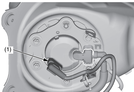
(1) connettore della pompa del carburante
