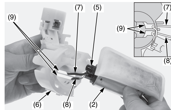
(2) gruppo della pompa del carburante (7) filo giallo (8) filo verde (5) O-ring (nuovo) (9) scanalature (6) supporto dell'unità della pompa del carburante
