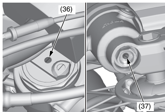
(36) registro dello smorzamento della compressione (37) registro dello smorzamento dell'espansione
