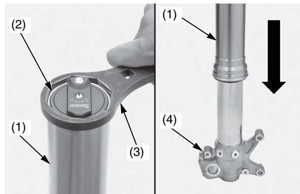
(1) tubo esterno (2) gruppo del pompante forcella
