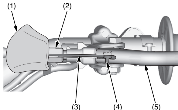
(1) parapolvere (2) registro (3) cavo della frizione (4) estremità del cavo della frizione (5) leva della frizione
