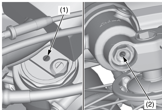
(1) vite di regolazione dello smorzamento della compressione
