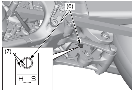
(6) registro dello smorzamento dell'estensione (7) segni punzonati
