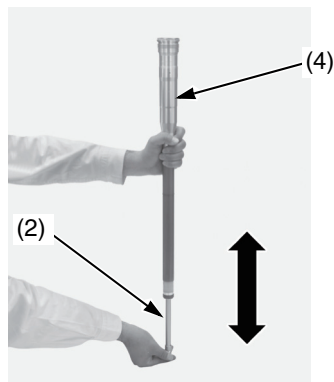
(2) asta del pompante forcella (4) gruppo del pompante della forcella
