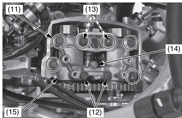
(11) bulloni A del supporto dell'albero a camme (12) bulloni B del supporto dell'albero a camme (13) rondelle (14) bullone di fermo dell'albero dei bilancieri (15) supporto dell'albero a camme
