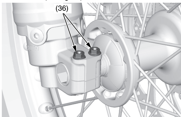
(36) bulloni di fissaggio del perno ruota destro
