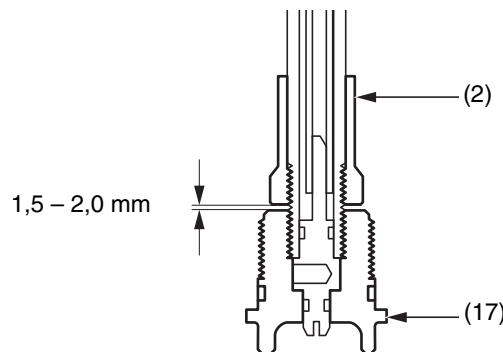
(2) dado di bloccaggio del bullone centrale della forcella (17) bullone centrale della forcella
