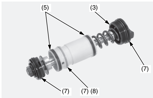
(3) gruppo bulloni della forcella (5) boccole dei bulloni della forcella (7) O-ring (nuovi) (8) fascia elastica del pistone (nuova)
