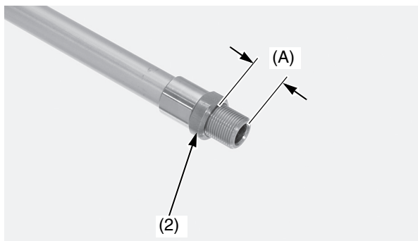
(2) dado di bloccaggio del bullone centrale della forcella (A) lunghezza della filettatura
