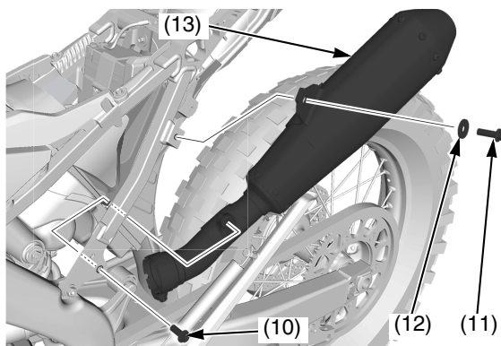
(10) bullone di fissaggio A del terminale di scarico sinistro
