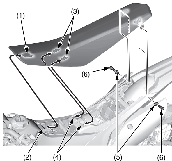
(1) sporgenza anteriore della sella (2) scanalatura (3) sporgenze centrali della sella (4) scanalature della base di supporto della sella (5) collari (6) bulloni di fissaggio della sella
