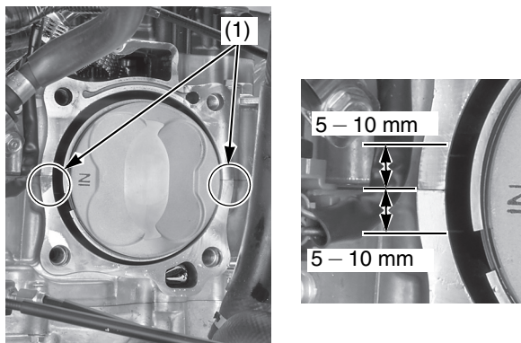
(1) superficie di accoppiamento del cilindro
