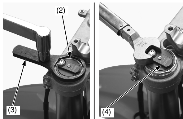
(2) gruppo del pompante forcella (3) chiave inglese (4) gruppo bulloni della forcella
