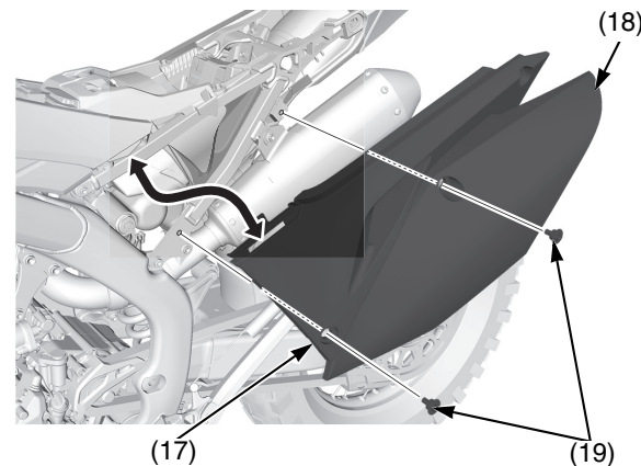
(17) coperchi dell'alloggiamento del filtro dell'aria (18) coperture laterali (19) bulloni
