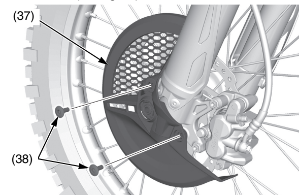
(37) coperchio del disco (38) viti a brugola del coperchio del disco
