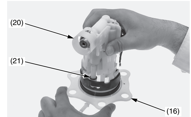
(16) base della pompa del carburante (20) gruppo del supporto dell'unità della pompa del carburante (21) O-ring
