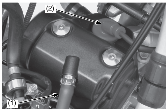
(1) tubo di sfiato
