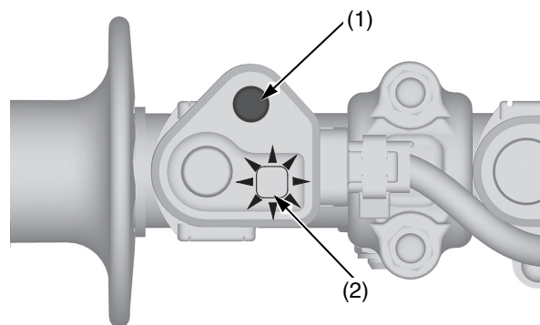
(1) pulsante di selezione settaggio motore (2) spia del settaggio motore (blu)
