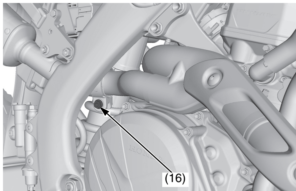
(16) bullone del morsetto del terminale di scarico destro
