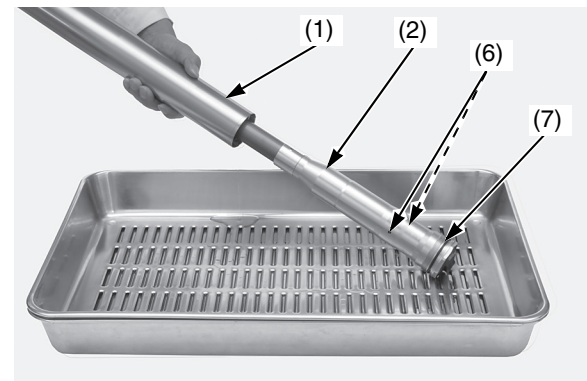
(1) tubo esterno (2) gruppo del pompante forcella (6) fori dell'olio (7) O-ring
