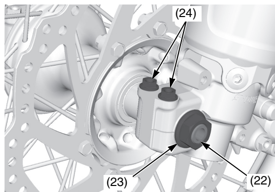
(22) perno dell'asse anteriore (23) dado del perno ruota anteriore (24) bulloni di fissaggio del perno ruota sinistro
