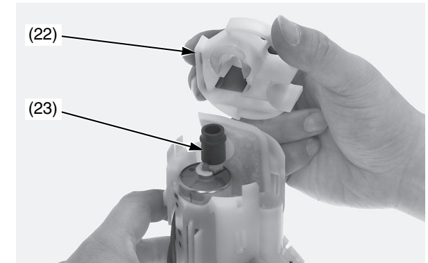
(22) fermo della pompa del carburante (23) tampone ammortizzatore
