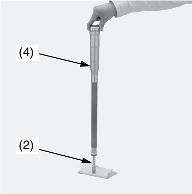
(2) asta del pistone del pompante forcella (4) gruppo del pompante della forcella
