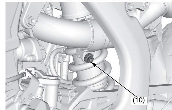
(10) bullone del morsetto del terminale di scarico sinistro
