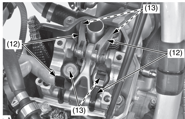
(12) bilancieri (13) spessori
