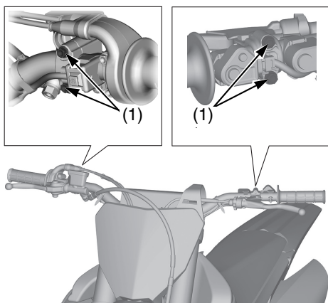
(1) bulloni di fissaggio delle leve di comando
