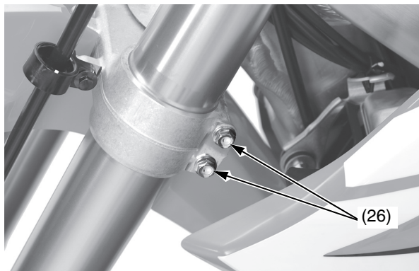
(26) bulloni di fissaggio inferiori del ponte della forcella
