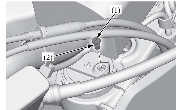
(1) vite di scarico della pressione (2) O-ring (nuovo)
