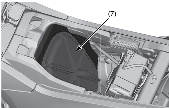
(7) alloggiamento del filtro dell'aria
