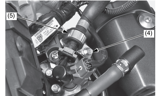
(4) bullone (5) morsetto e gommino di posizionamento
