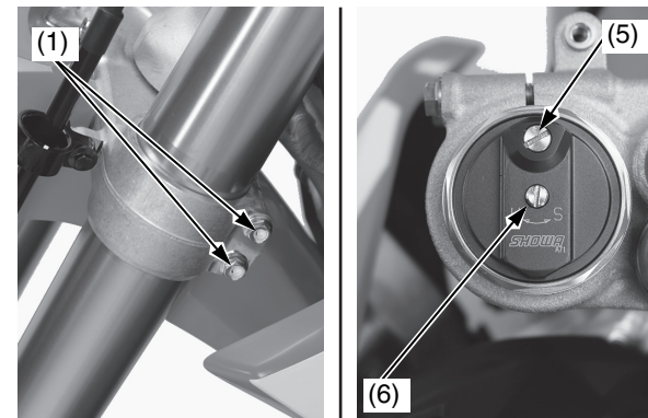
(1) bulloni di fissaggio inferiori del ponte della forcella (5) vite di scarico della pressione (6) registro dello smorzamento della compressione
