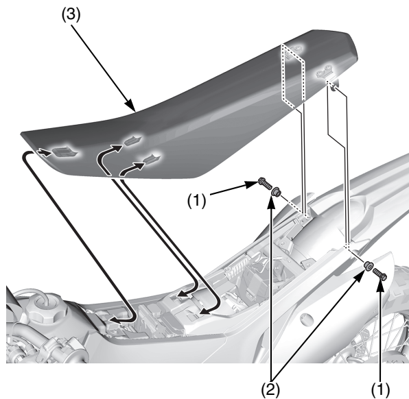
(1) bulloni di fissaggio della sella (3) sella (2) collari
