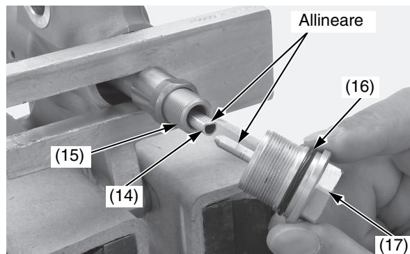
(14) asta pompante (15) asta del pistone (16) O-ring (nuovo) (17) bullone centrale della forcella
