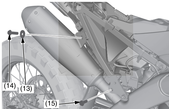
(13) rondella (14) bullone di fissaggio B del terminale di scarico destro (15) bullone di fissaggio A del terminale di scarico destro
