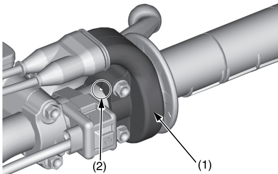
(1) alloggiamento dell'acceleratore (2) punto verniciato
