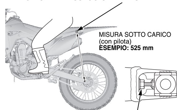
DADO DI BLOCCAGGIO DEL REGISTRO DELLA CATENA
