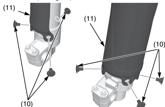
(10) viti a brugola dell'elemento di protezione della forcella (11) elementi di protezione della forcella
