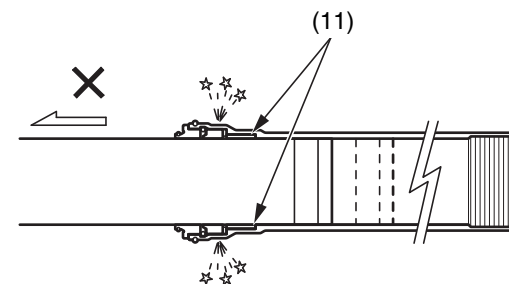
(11) boccola guida
