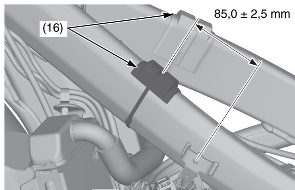
(16) tamponi di gomma
