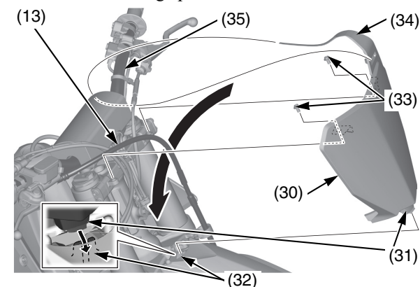
(13) tubo flessibile del freno (33) bulloni (30) targa (34) linguetta della targa (31) linguetta (35) manubrio (32) fessura
