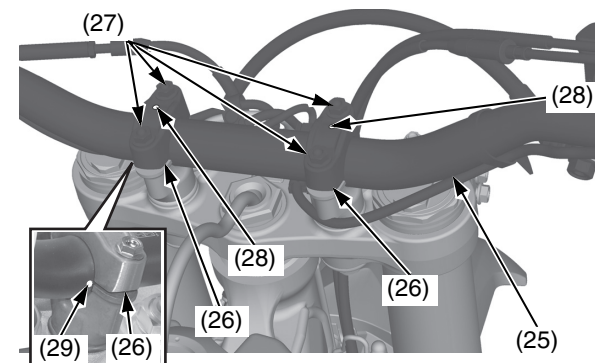
(25) manubrio (26) supporti superiori del manubrio (27) bulloni dei supporti superiori del manubrio (28) punzonatura (29) punto verniciato
