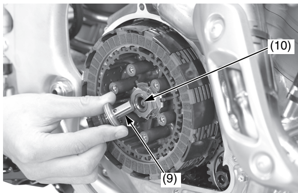
(9) spingidisco della frizione (10) asta spingidisco della frizione
