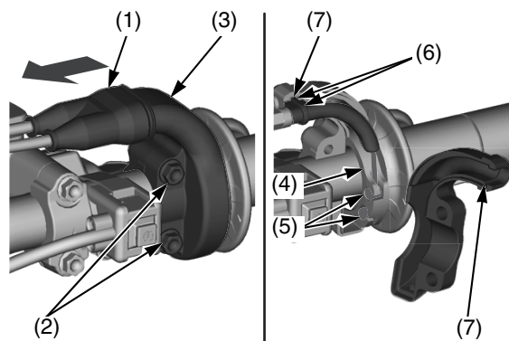
(1) alloggiamento dell'acceleratore (2) punto verniciato
