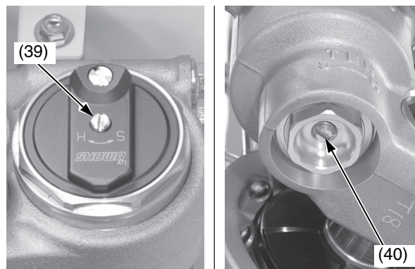
(39) registro dello smorzamento della compressione (40) registro dello smorzamento dell'estensione
