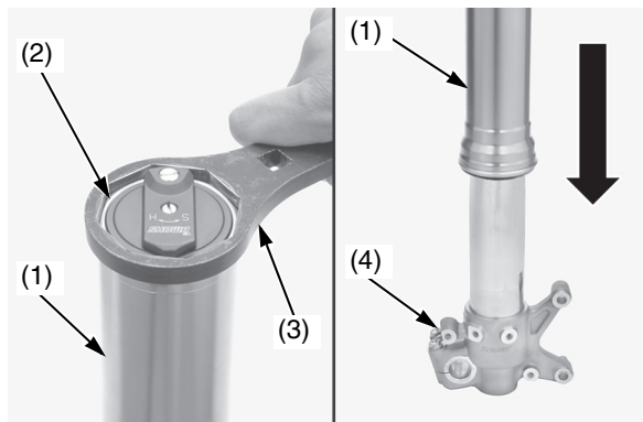
(1) tubo esterno (2) gruppo del pompante forcella (3) chiave inglese (4) supporto dell'asse
