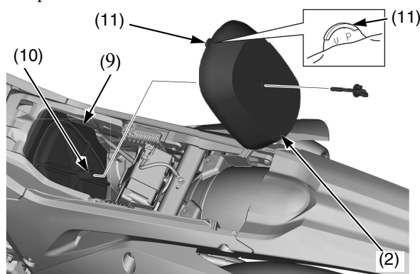
(2) gruppo del filtro dell'aria (9) superficie di contatto (10) supporto dell'alloggiamento del filtro dell'aria (11) linguetta del segno "UP"
