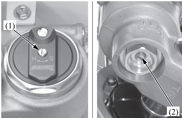
(1) registro dello smorzamento della compressione (2) registro dello smorzamento dell'estensione
