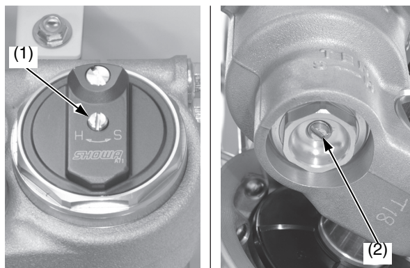
(1) vite del registro dello smorzamento della compressione
