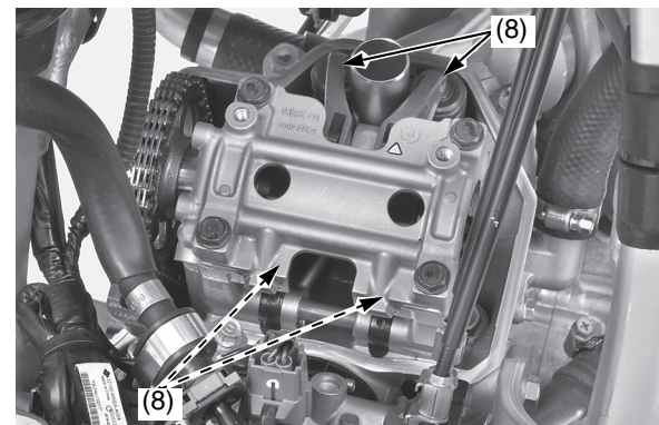
(8) bilancieri
