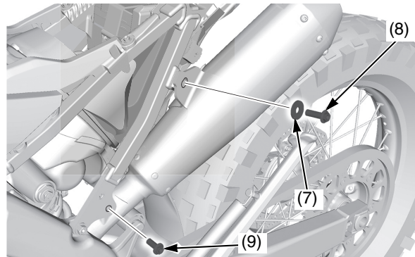
(7) rondella
