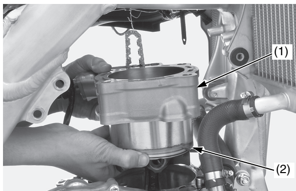
(1) cilindro (2) pistone
