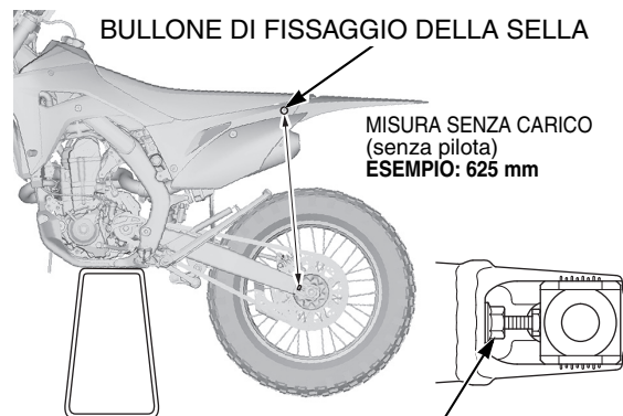
DADO DI BLOCCAGGIO DEL REGISTRO DELLA CATENA
