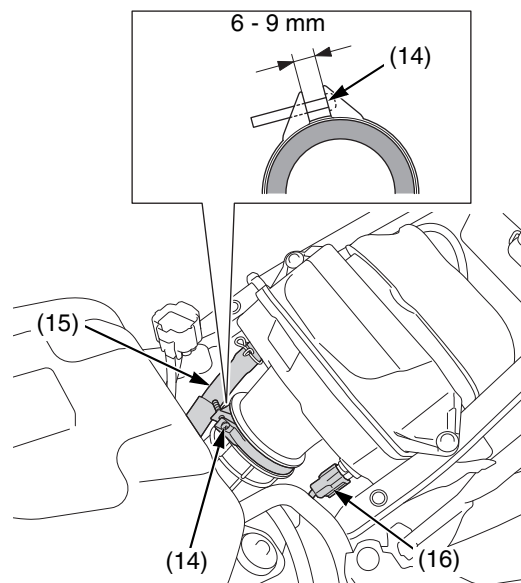
(14) vite del morsetto del tubo di collegamento del filtro dell'aria (15) tubo di sfiato (16) connettore del sensore IAT
