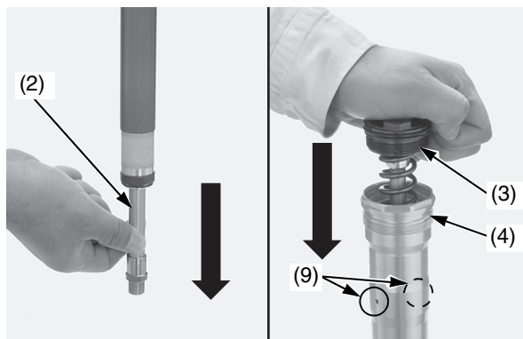
(2) asta del pistone del pompante forcella (3) gruppo bulloni della forcella (4) gruppo del pompante della forcella (9) fori dell'olio
