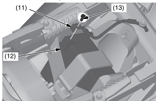
(11) terminale negativo (-) (12) batteria (13) bullone del terminale negativo (-)
