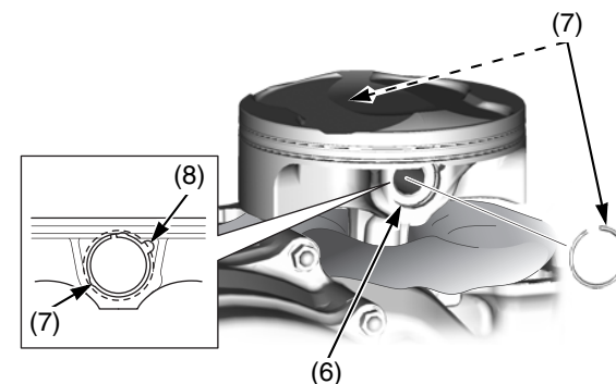
(6) spinotto del pistone (7) fermagli dello spinotto del pistone (nuovi) (8) cavità del pistone
