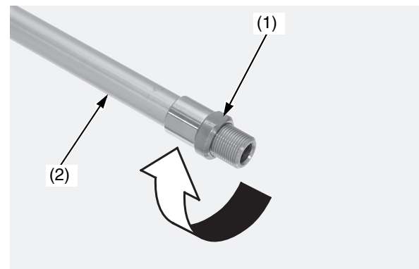
(1) dado di bloccaggio del bullone centrale della forcella (2) asta del pistone del pompante forcella
