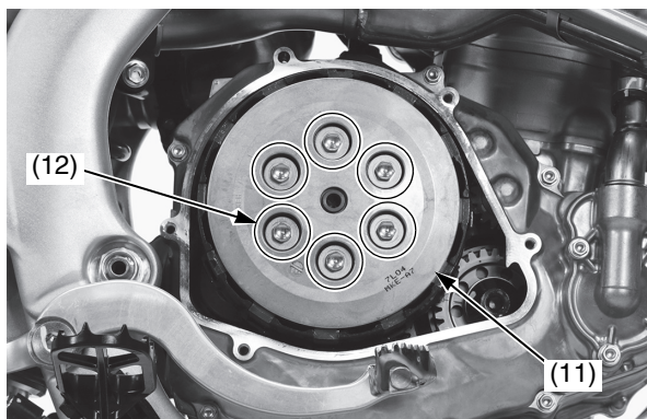
(11) piastra spingidisco della frizione (12) molle e bulloni della frizione
