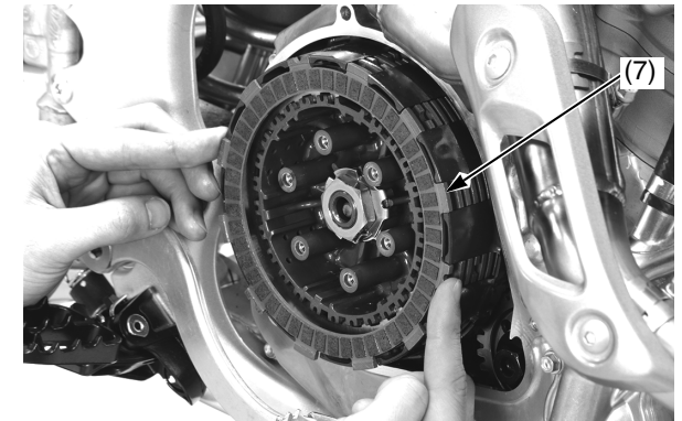
(7) dischi conduttori, dischi condotti della frizione, molla antivibrazioni e sede della molla
