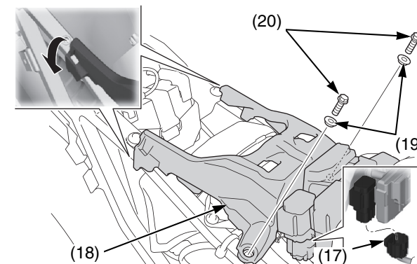
(17) connettore del relè motorino di avviamento/accensione (18) base di supporto della sella (19) collari (20) bulloni di fissaggio della base di supporto della sella
