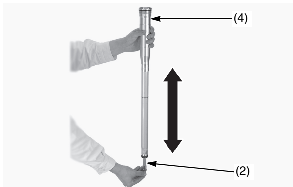
(2) asta del pistone del pompante forcella (4) gruppo del pompante della forcella
