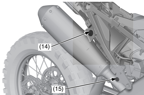
(14) bullone di fissaggio B del terminale di scarico destro (15) bullone di fissaggio A del terminale di scarico destro
