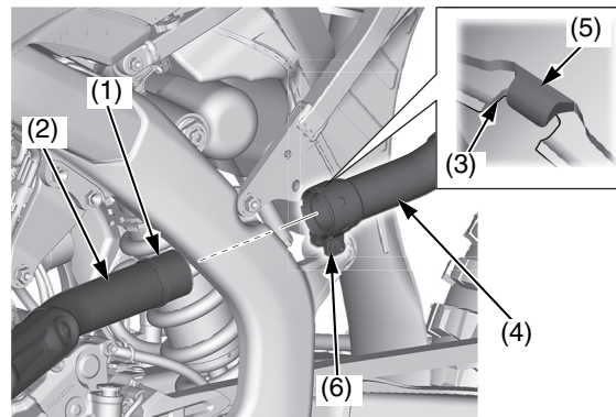
(1) guarnizione (2) collettore di scarico (3) cavità (4) terminale di scarico sinistro (5) linguetta (6) morsetto del terminale di scarico sinistro
