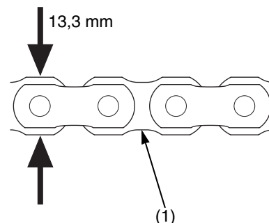
(1) piastrina (interna) della catena di trasmissione
