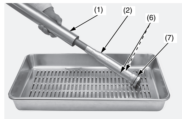
(1) tubo esterno (2) gruppo del pompante forcella (6) fori dell'olio (7) O-ring
