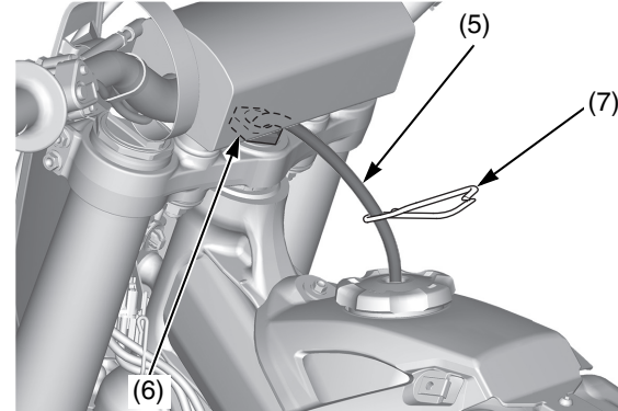
(5) tubo di sfiato (6) dado del piantone dello sterzo
