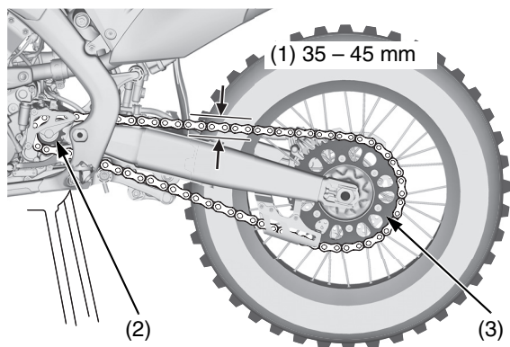
(1) gioco della catena di trasmissione (3) ingranaggio condotto (2) ingranaggio conduttore
