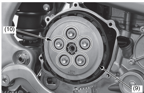
(9) piastra spingidisco della frizione (10) molle della frizione e bulloni
