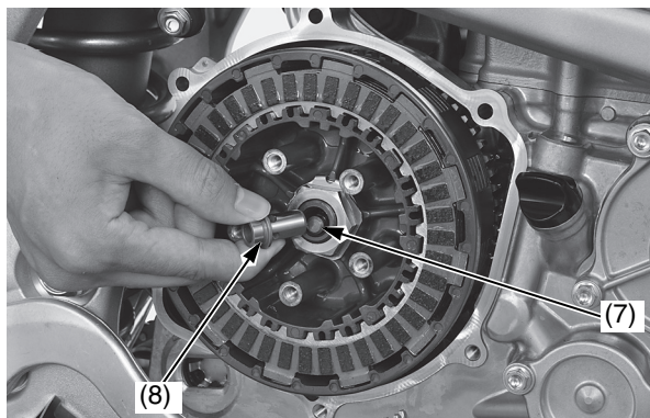
(7) asta spingidisco della frizione (8) spingidisco della frizione
