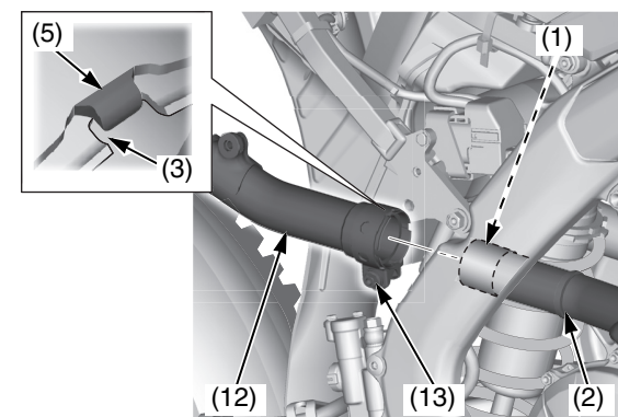
(1) guarnizione (2) collettore di scarico (3) cavità (5) linguetta (12) terminale di scarico destro (13) morsetto del terminale di scarico destro
