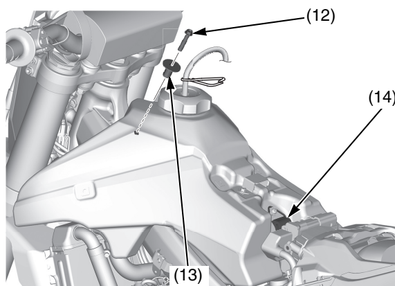
(12) bullone del serbatoio carburante (14) fascia del serbatoio del carburante (13) collare
