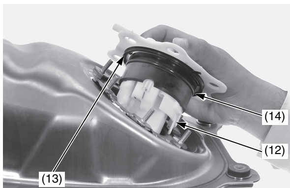
(12) unità della pompa del carburante (14) O-ring (13) parapolvere
