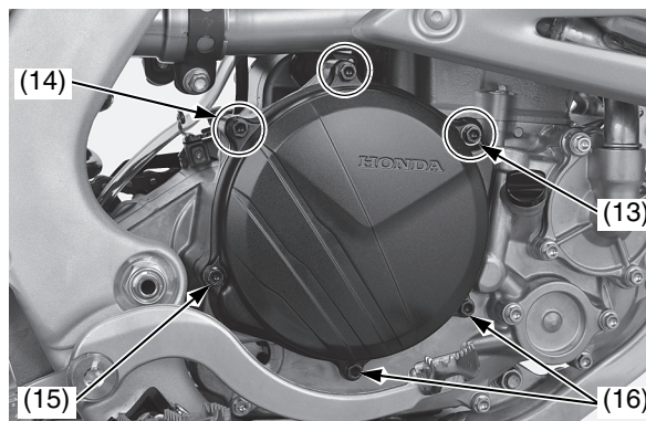
(13) rondella (nuova) (14) bulloni A del coperchio della frizione (15) bullone B del coperchio della frizione (16) bulloni C del coperchio della frizione
