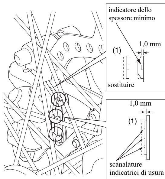
(1) pastiglie del freno
