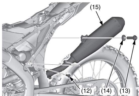
(12) bullone di fissaggio A del terminale di scarico sinistro (13) bullone di fissaggio B del terminale di scarico sinistro (14) rondella (15) terminale di scarico sinistro
