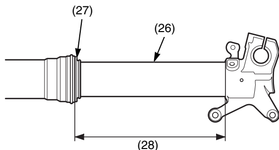
(26) superficie di scorrimento (27) parapolvere della forcella (28) lunghezza
