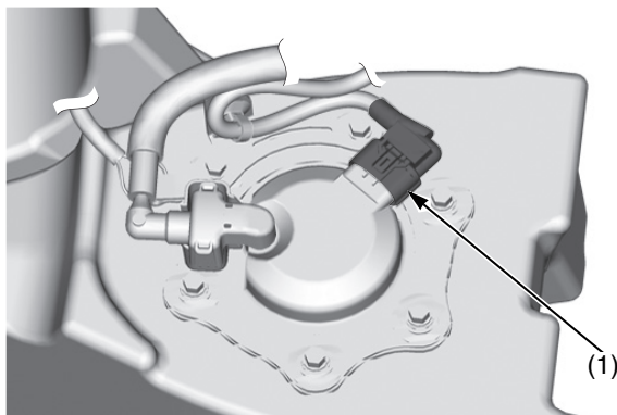
(1) connettore della pompa del carburante
