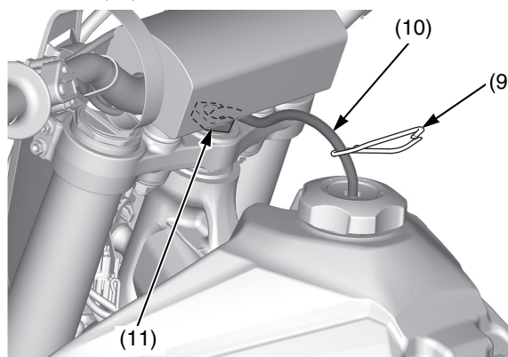
(9) morsetto stringitubo (11) dado del piantone dello sterzo (10) tubo di sfiato
