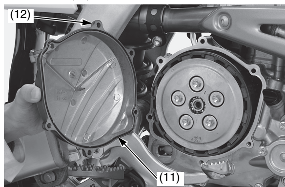
(11) O-ring (nuovo) (12) coperchio della frizione
