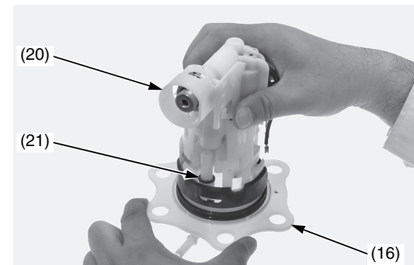
(16) base della pompa del carburante (20) gruppo del supporto dell'unità della pompa del carburante (21) O-ring
