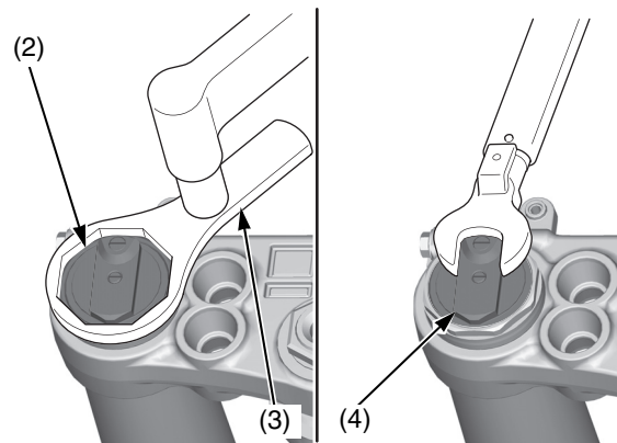
(2) gruppo del pompante forcella (3) chiave inglese (4) gruppo bulloni della forcella
