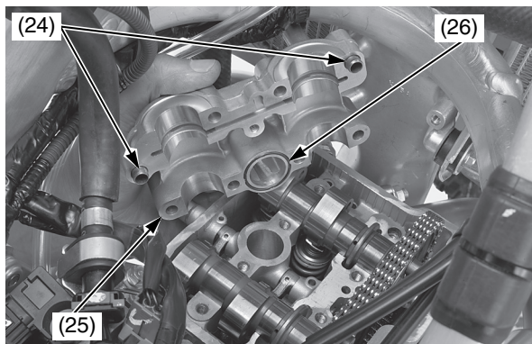
(24) perni di centraggio (25) supporto dell'albero a camme (26) O-ring (nuovo)
