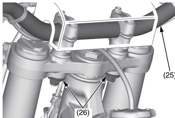
(25) manubrio (26) gommini di montaggio, rondelle e dadi dei supporti inferiori del manubrio
