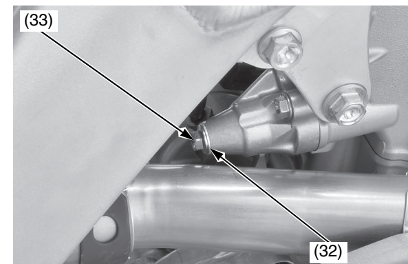
(32) rondella di tenuta (nuova) (33) bullone del coperchio del sollevatore del tenditore della catena di distribuzione
