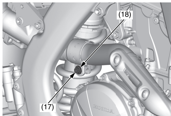
(17) bullone del morsetto del terminale di scarico destro (18) rondella
