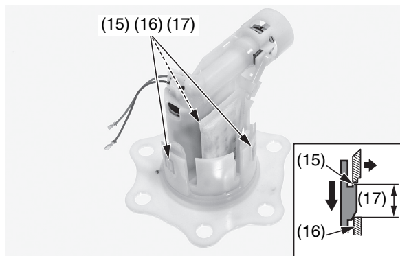
(15) ganci (16) linguette
