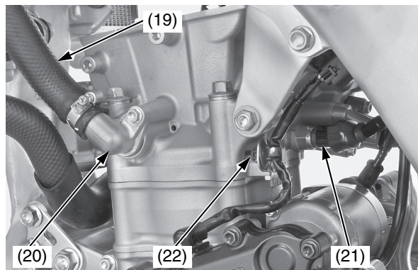
(19) tubo flessibile sinistro del radiatore (20) giunto sinistro del tubo flessibile dell'acqua (21) connettore del sensore ECT (22) fermaglio della fascetta del cablaggio
