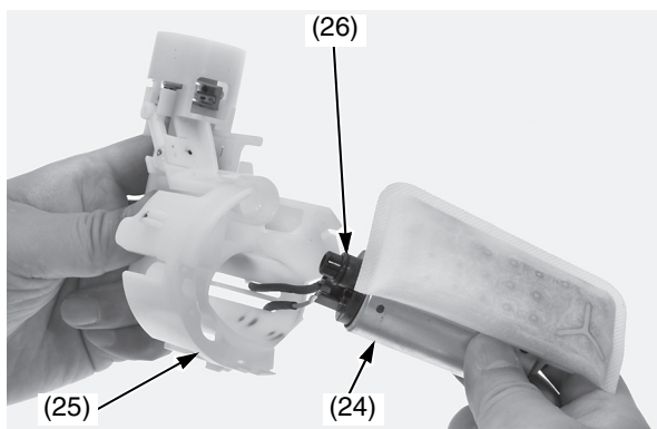
(24) gruppo della pompa del carburante (25) supporto dell'unità della pompa del carburante (26) O-ring
