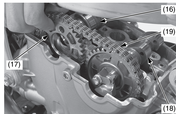
(16) albero a camme di aspirazione (17) ruota dentata della distribuzione di aspirazione (18) albero a camme di scarico (19) catena di distribuzione
