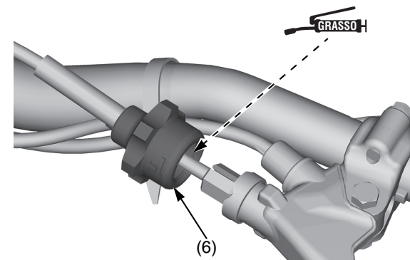
(6) registro all'estremità del cavo della frizione
