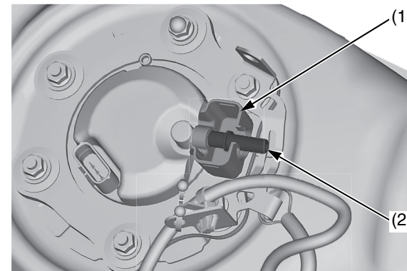
(1) coperchio di gomma (2) giunto del carburante
