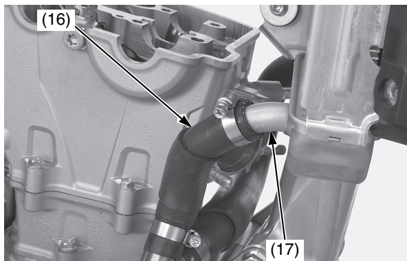
(16) tubo flessibile destro del radiatore (17) giunto del tubo flessibile destro del radiatore
