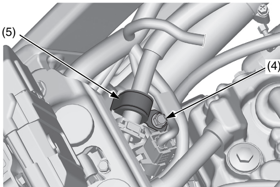
(4) bullone (5) morsetto e gommino di posizionamento
