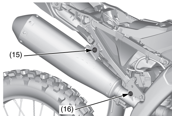
(15) bullone di fissaggio B del terminale di scarico destro (16) bullone di fissaggio A del terminale di scarico destro
