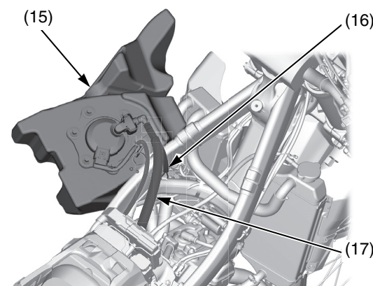
(15) serbatoio del carburante (16) cavo del fermo del serbatoio del carburante (17) tubo di alimentazione del carburante
