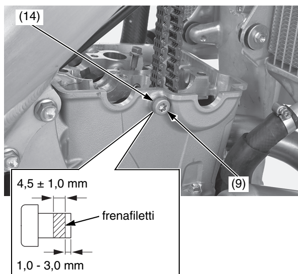
(9) bullone di tenuta (14) rondella di tenuta (nuova)
