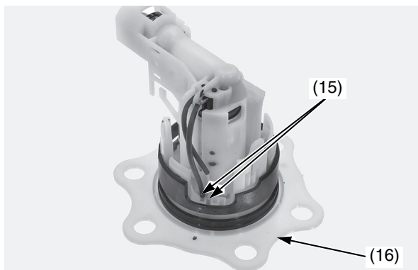
(15) terminali dei fili della pompa del carburante (16) base della pompa del carburante
