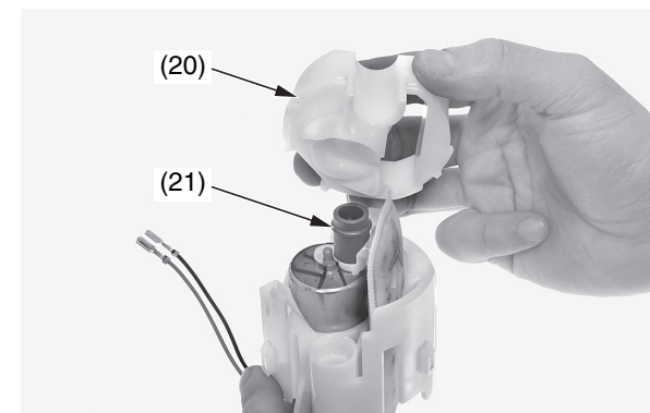
(20) fermo della pompa del carburante (21) tampone ammortizzatore
