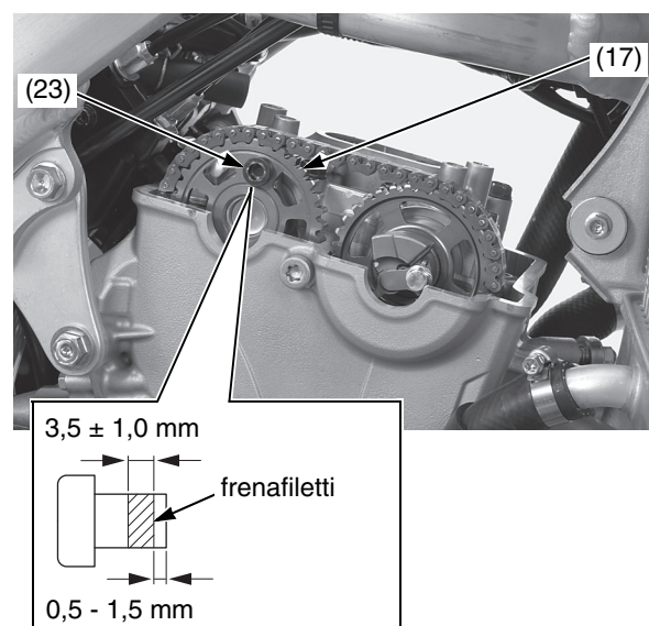
(17) ruota dentata della distribuzione di aspirazione (23) bullone della ruota dentata della distribuzione
