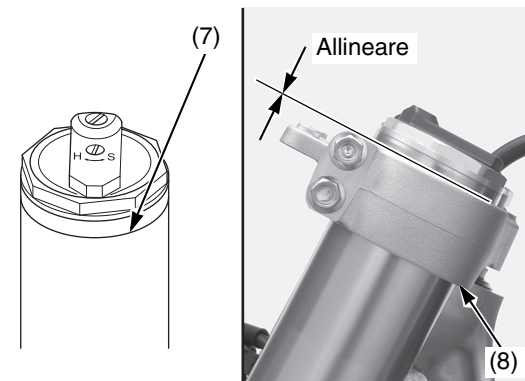
(7) scanalatura (8) ponte superiore della forcella
