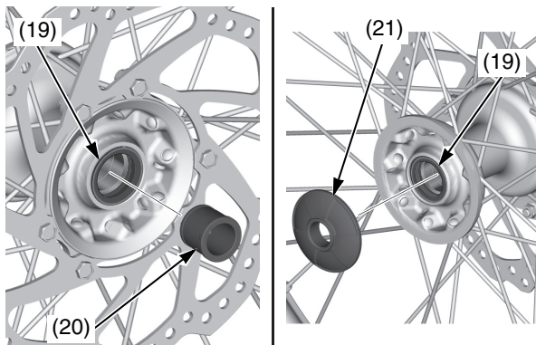
(19) labbri del parapolvere (21) collare destro (20) collare sinistro
