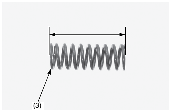
(3) molla della frizione
