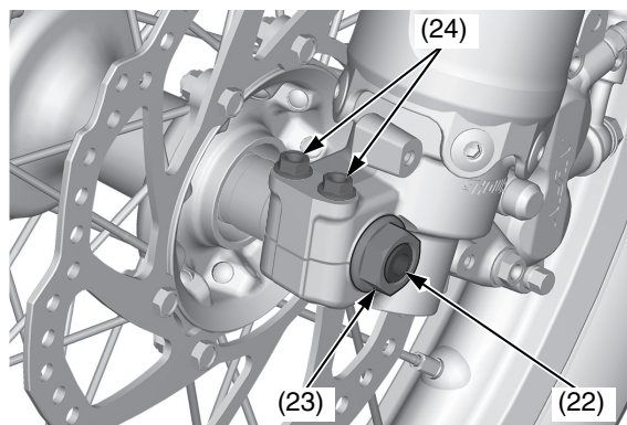
(22) perno dell'asse anteriore (23) dado del perno ruota anteriore (24) bulloni di fissaggio del perno ruota sinistro
