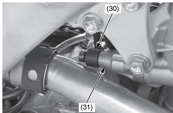
(30) attrezzo di blocco del tenditore (31) sollevatore del tenditore della catena di distribuzione
