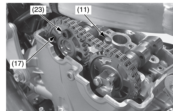
(11) bullone di fermo dell'albero dei bilancieri (17) ruota dentata della distribuzione di aspirazione (23) bullone della ruota dentata della distribuzione
