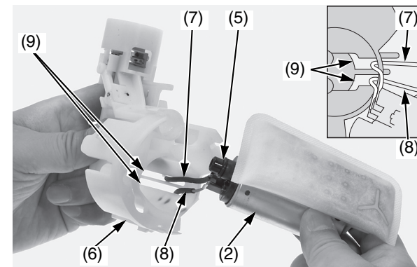
(2) gruppo della pompa del carburante (7) filo giallo (5) O-ring (nuovo) (8) filo verde (6) supporto dell'unità della pompa del carburante (9) scanalature carburante
