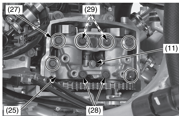
(11) bullone di fermo dell'albero dei bilancieri (25) supporto dell'albero a camme (27) bulloni A del supporto dell'albero a camme (28) bulloni B del supporto dell'albero a camme (29) rondelle (nuove)
