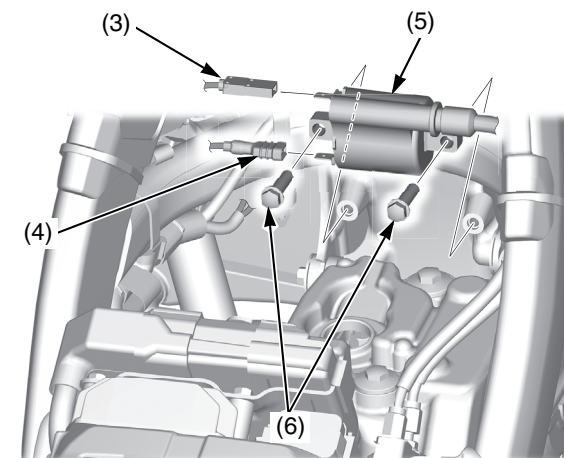
(3) connettore A della bobina di accensione (5) bobina di accensione (4) connettore B della bobina di accensione (6) bulloni della bobina di accensione
