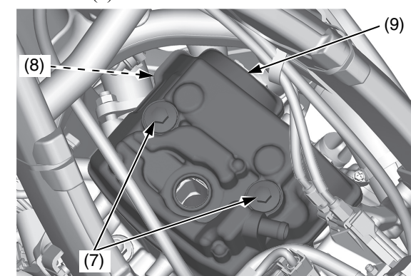
(7) viti a brugola del coperchio della testata, guarnizioni di gomma (8) guarnizione del coperchio della testata (9) coperchio della testata
