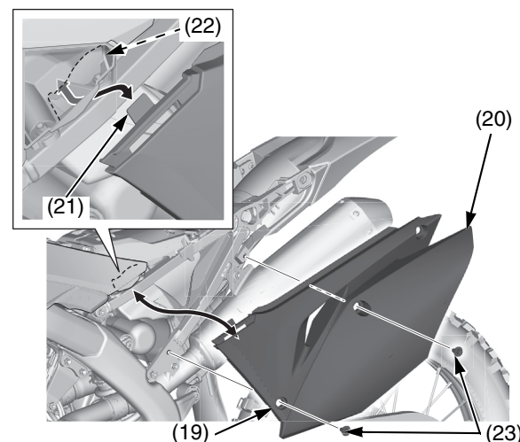
(19) coperchio dell'alloggiamento del filtro dell'aria (20) copertura laterale (21) linguetta del coperchio dell'alloggiamento del filtro dell'aria (22) scanalatura della base di supporto della sella (23) bulloni
