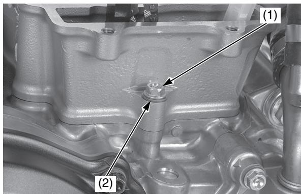
(1) bullone del cilindro (2) rondella di tenuta
