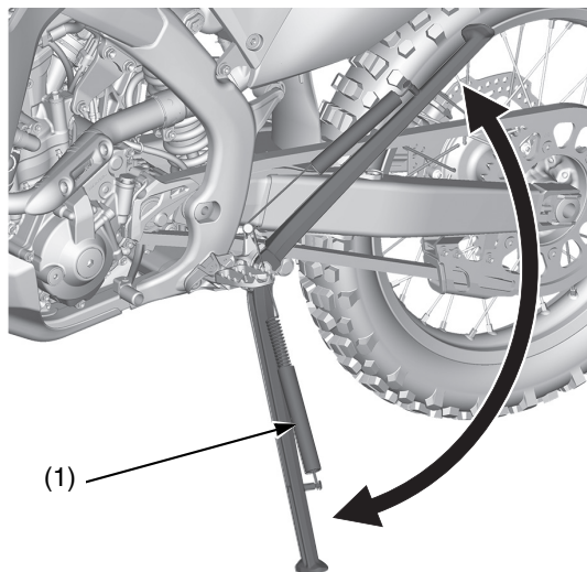
(1) molla del cavalletto laterale
