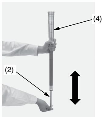
(2) asta del pistone pompante forcella (4) gruppo del pompante della forcella
