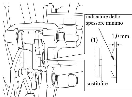
(1) pastiglie del freno
