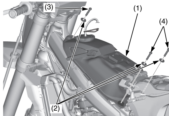
(1) serbatoio del carburante (2) rondelle
