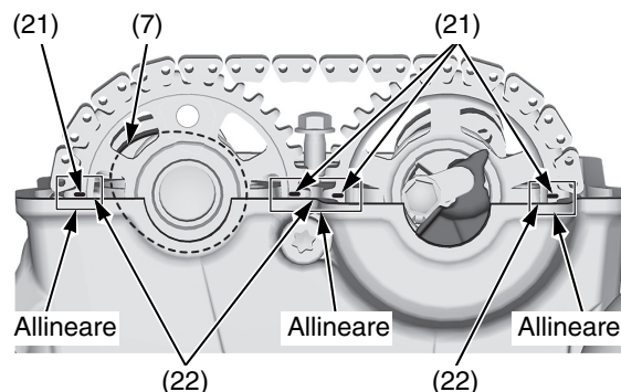
(7) lobo della camma dell'albero a camme (21) segni della fasatura (22) superficie di accoppiamento della testata
