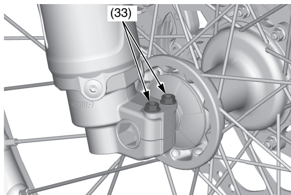
(33) bulloni di fissaggio del perno ruota destro
