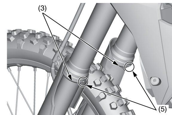
(3) anelli di usura
