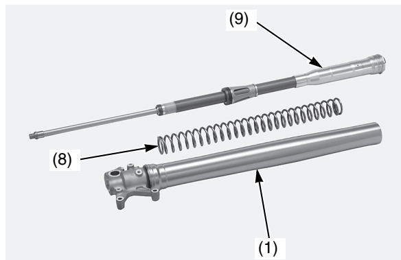
(1) gruppo della forcella (9) gruppo del pompante della forcella (8) molla della forcella
