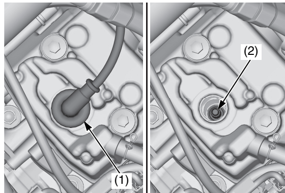
(1) cappuccio della candela (2) candela
