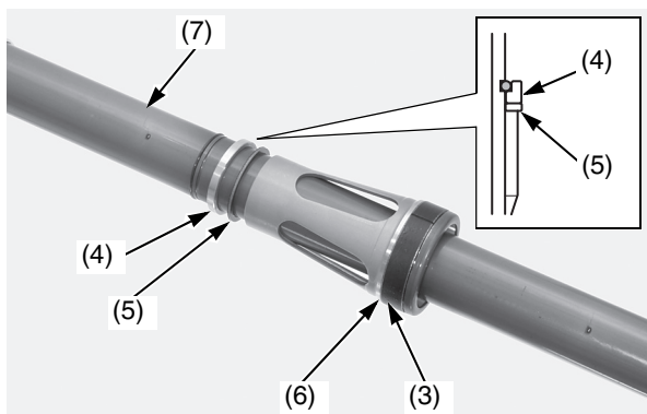
(3) boccia di scorrimento (6) collare della sede della molla (4) fermo della sede (5) anello di sostegno (7) pompante della forcella
