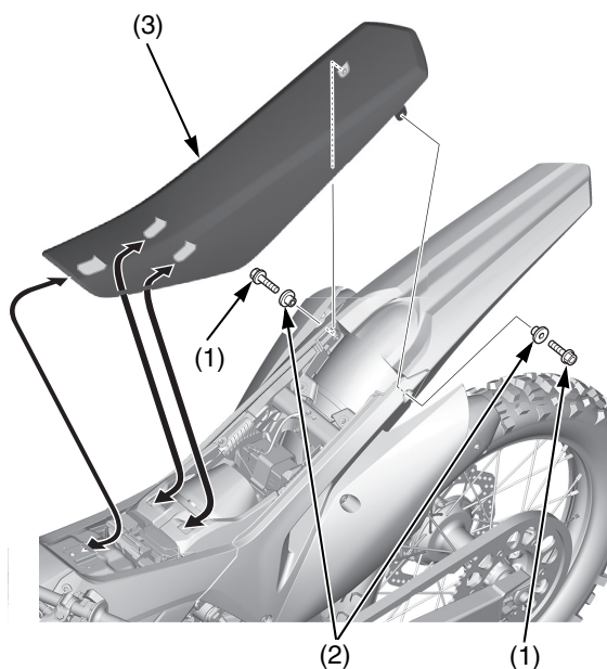
(1) bulloni di fissaggio della sella (3) sella (2) collari
