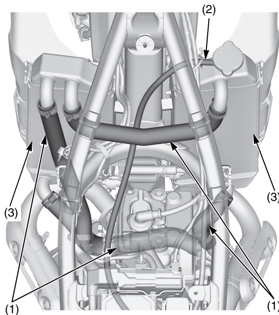
(1) tubi flessibili del radiatore (3) alette del radiatore (2) tubo flessibile di trabocco
