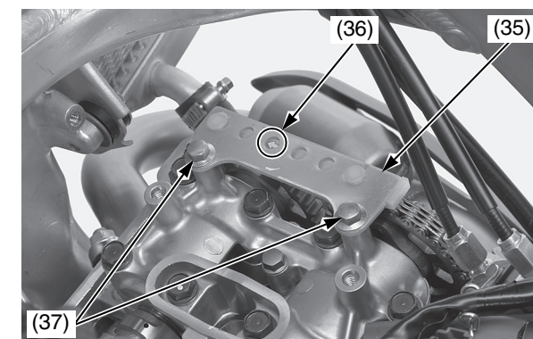
(35) guida della catena di distribuzione (36) segno "↔"
