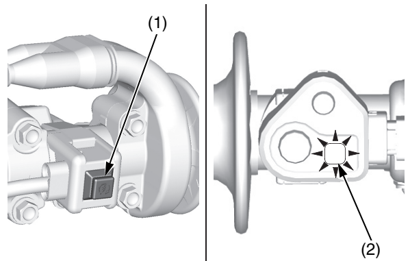
(1) pulsante di avviamento (2) spia del sistema di controllo lancio (viola)
