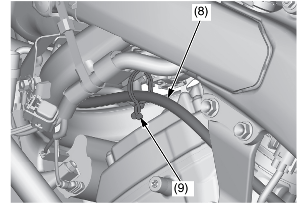
(8) tubo flessibile di trabocco (9) morsetto
