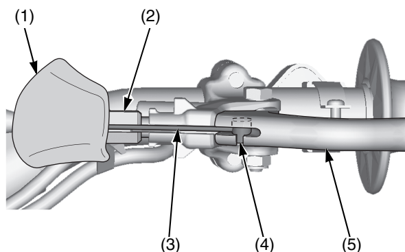
(1) parapolvere (2) registro (3) cavo della frizione (4) estremità del cavo della frizione (5) leva della frizione
