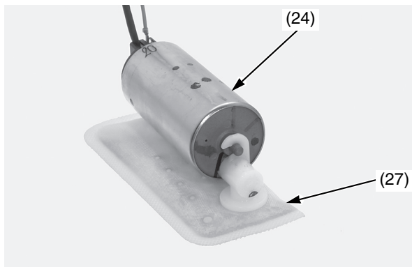
(24) gruppo della pompa del carburante (27) filtro della pompa del carburante
