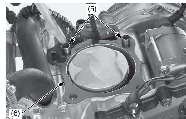
(5) perni di centraggio
