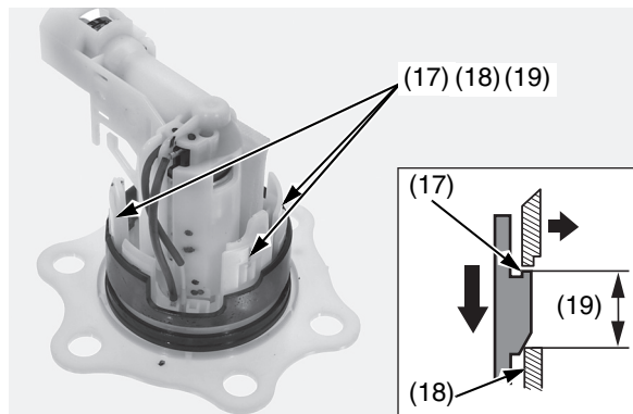
(17) ganci (18) linguette
