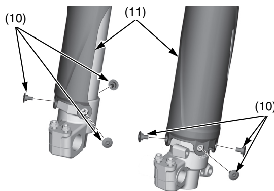
(10) viti a brugola dell'elemento di protezione della forcella (11) elementi di protezione della forcella
