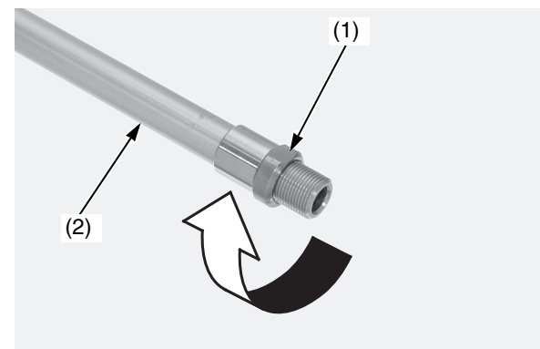
(1) dado di bloccaggio del bullone centrale della forcella (2) asta del pistone pompante forcella
