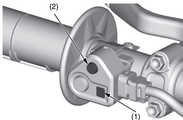
(1) spia del settaggio motore (blu) (2) pulsante di selezione settaggio motore
