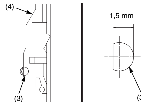
(3) anello di usura
