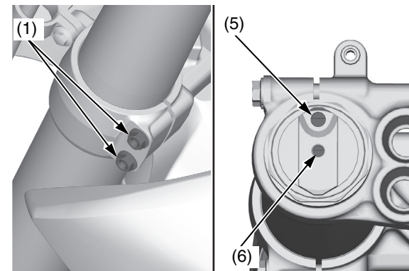
(1) bulloni di fissaggio inferiori del ponte della forcella (5) vite di scarico della pressione dell'aria (6) registro dello smorzamento della compressione
