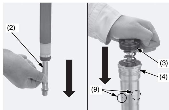
(2) asta del pistone pompante forcella (3) gruppo bulloni della forcella (4) gruppo del pompante della forcella (9) fori dell'olio
