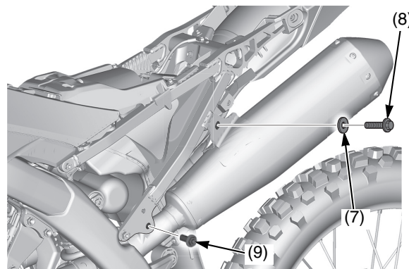
(7) rondella (8) bullone di fissaggio B del terminale di scarico sinistro (9) bullone di fissaggio A del terminale di scarico sinistro
