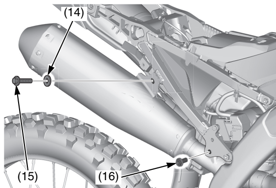
(14) rondella (15) bullone di fissaggio B del terminale di scarico destro (16) bullone di fissaggio A del terminale di scarico destro
