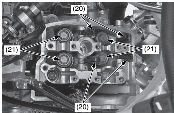
(20) bilancieri (21) spessori
