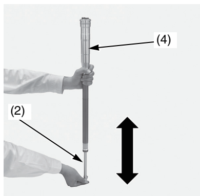
(2) asta del pistone pompante forcella
