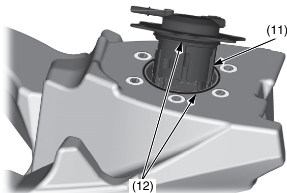
(11) unità della pompa del carburante (12) O-ring
