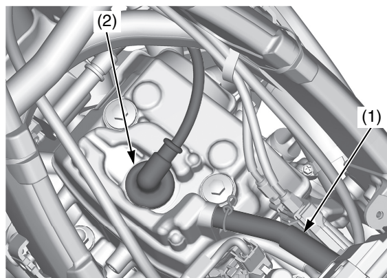
(1) tubo di sfiato (2) cappuccio della candela
