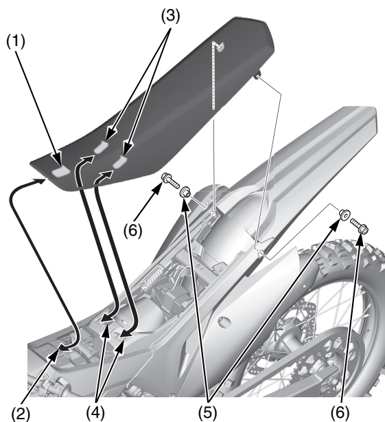
(1) sporgenza anteriore della sella (4) scanalature della base di supporto della sella (2) scanalatura (5) collari (3) sporgenze centrali della sella (6) bulloni di fissaggio della sella
