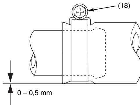
(18) vite del morsetto del tubo flessibile del radiatore
