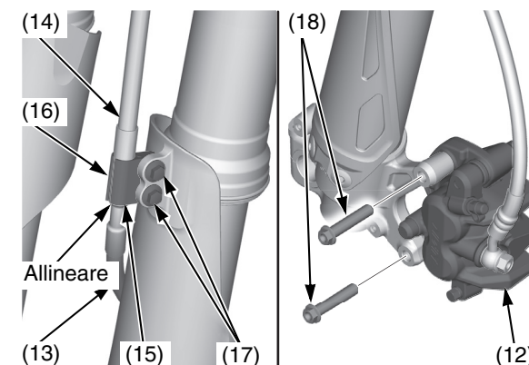
(12) pinza del freno (13) tubo flessibile del freno (14) protezione del tubo flessibile del freno (15) supporto A (16) supporto B (17) bulloni del morsetto del tubo flessibile del freno (18) bulloni di fissaggio della pinza del freno anteriore
