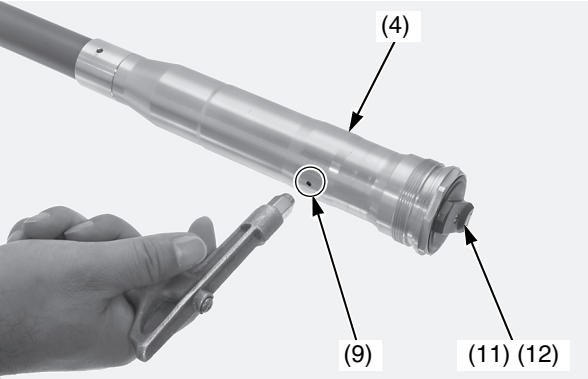
(4) gruppo del pompante della forcella (9) foro dell'olio (11) viti di scarico della pressione dell'aria (12) O-ring (nuovi)
