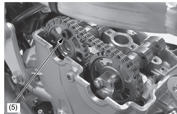
(5) bullone della ruota dentata della distribuzione
