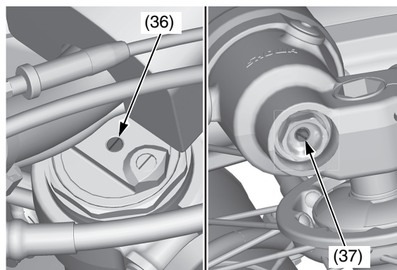
(36) registro dello smorzamento della compressione (37) registro dello smorzamento dell'estensione
