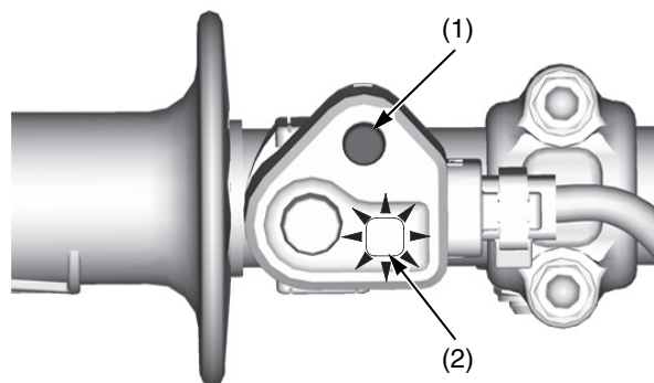
(1) pulsante di selezione settaggio motore (2) spia del settaggio motore (blu)
