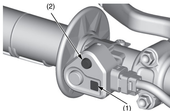
(1) spia del sistema di controllo lancio (viola) (2) pulsante di selezione settaggio motore
