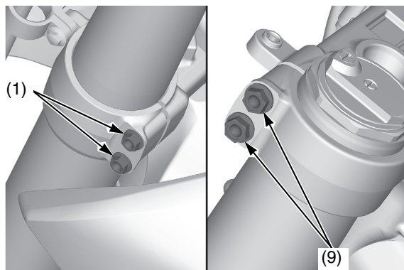
(1) bulloni di fissaggio inferiori del ponte della forcella (9) bulloni di fissaggio superiori del ponte della forcella
