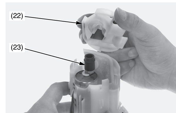
(22) fermo della pompa del carburante (23) tampone ammortizzatore
