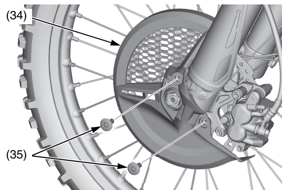
(34) coperchio del disco (35) viti a brugola del coperchio del disco
