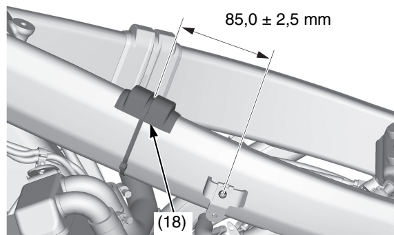
(18) tamponi di gomma
