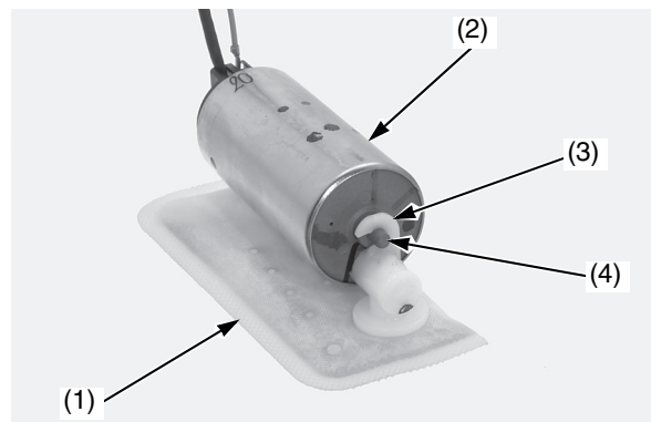
(1) filtro della pompa del carburante (3) gancio (2) gruppo della pompa del carburante (4) protuberanza di unione
