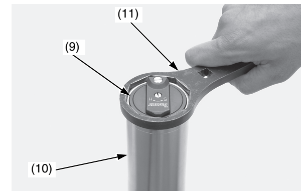
(9) gruppo del pompante della forcella (10) tubo esterno (11) chiave inglese
