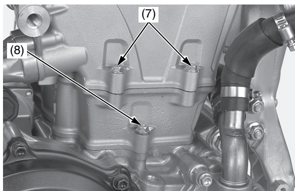
(7) bulloni della testata A (8) bullone del cilindro
