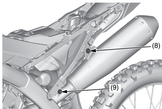
(8) bullone di fissaggio B del terminale di scarico sinistro (9) bullone di fissaggio A del terminale di scarico sinistro
