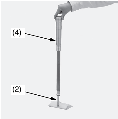
(2) asta del pistone pompante forcella (4) gruppo del pompante della forcella
