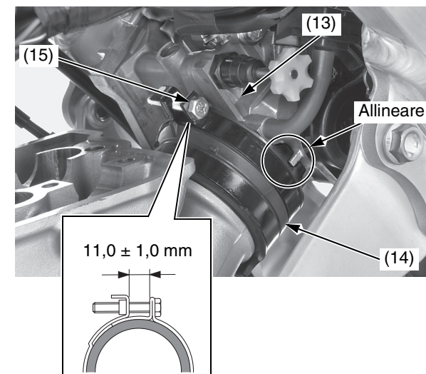
(13) corpo farfallato (14) isolatore
