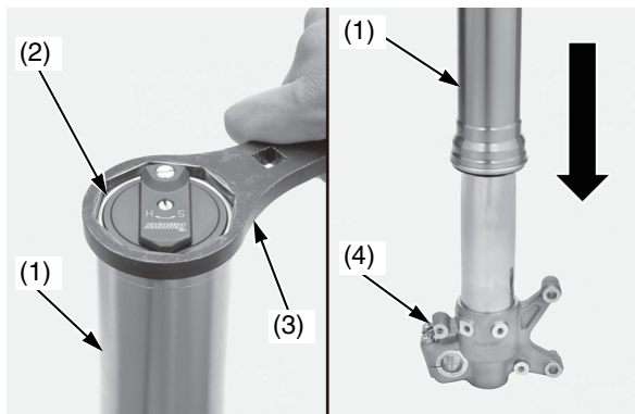
(1) tubo esterno (2) gruppo del pompante forcella (3) chiave inglese (4) supporto dell'asse
