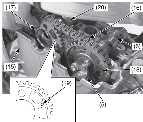
(5) peso del decompressore (6) albero a camme di scarico (15) testata (16) catena di distribuzione (17) ruota dentata della distribuzione di aspirazione (18) ruota dentata della distribuzione di scarico (19) segno "O" (20) albero a camme di aspirazione
