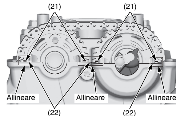
(21) segni della fasatura (22) superficie di accoppiamento della testata
