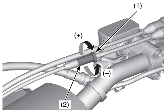
(1) dado di bloccaggio (2) registro (+) aumento del gioco (–) diminuzione del gioco
